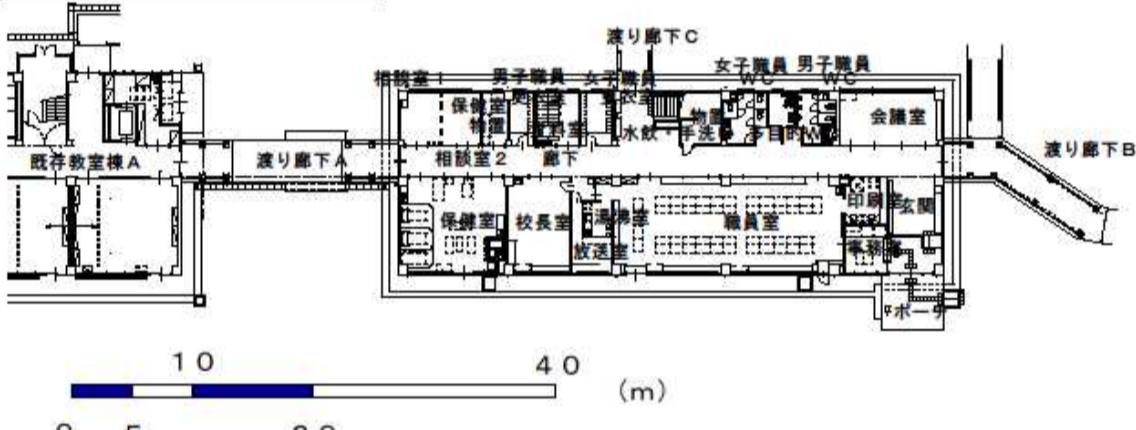
管理特別教室棟 1階平面図
