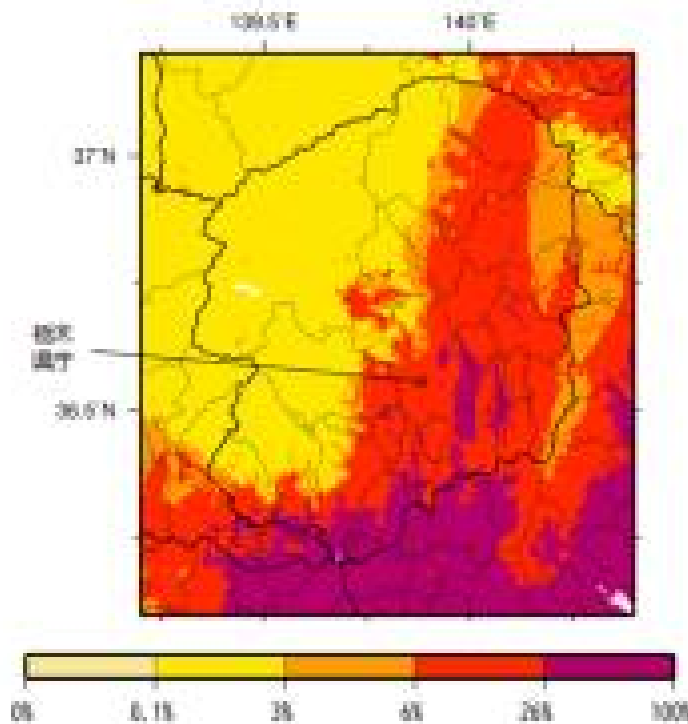
地震調査研究推進本部 「全国地震動予測地図 (2020年版)」から
