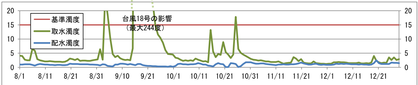
工水配水濁度計
