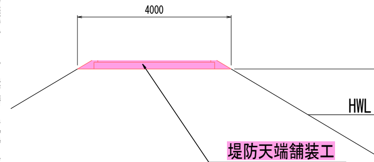
標準横断図
