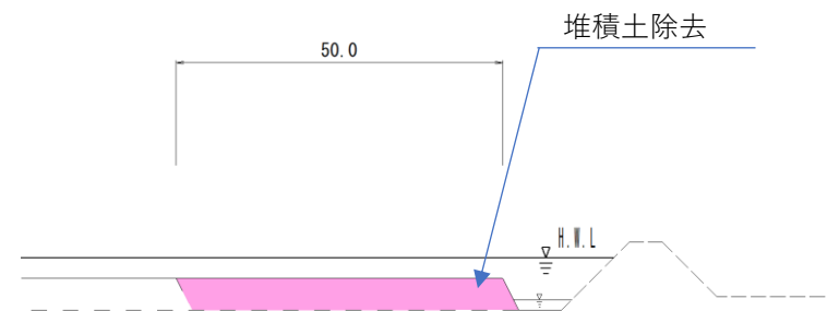
標準横断図
