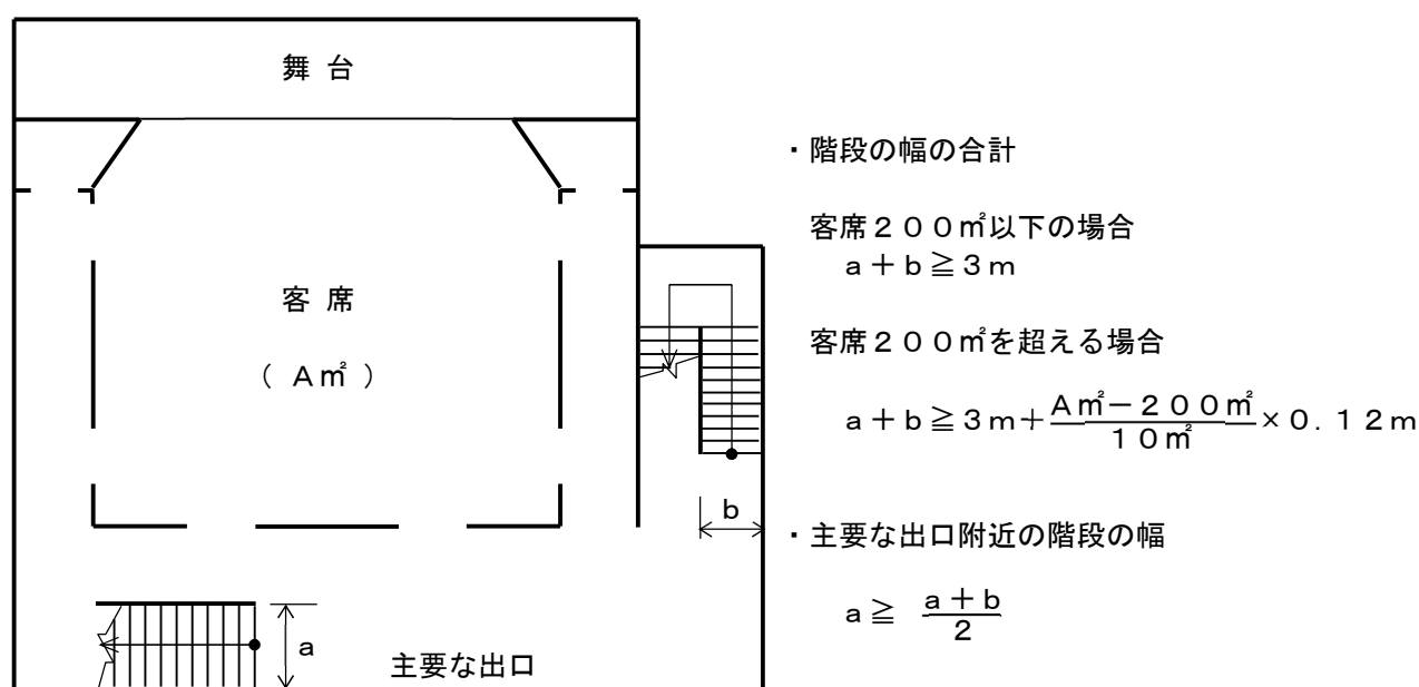
図5-16 階段の幅
