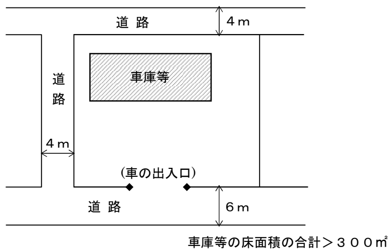
図5-46 敷地の出入口が接する道路の幅員
