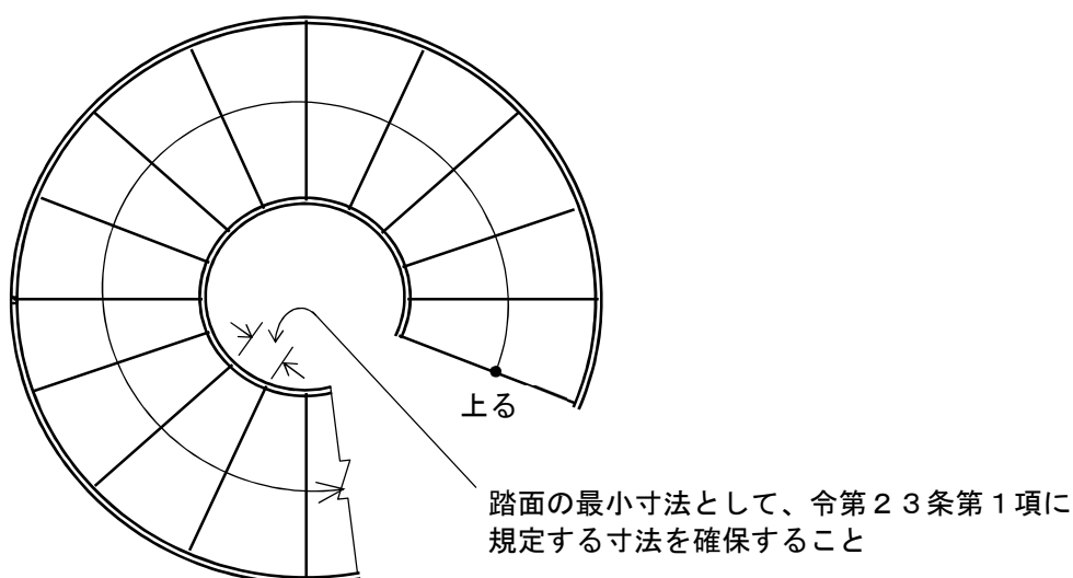
図5-6 らせん階段の寸法
