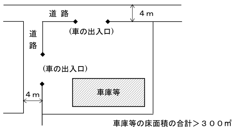
図5-47 敷地の出入口が2以上の道路に接する場合（第1号）
