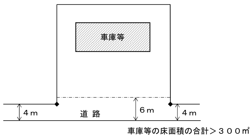
図5-48 敷地の一部が道路と一体となっている場合（第2号）
