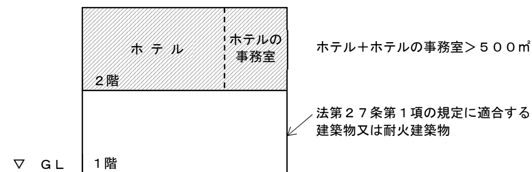
図5-26 ホテル等の一部に附属部分（事務室等）がある場合
