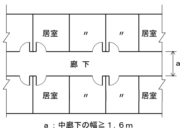
図5-44 両側に居室がある場合
