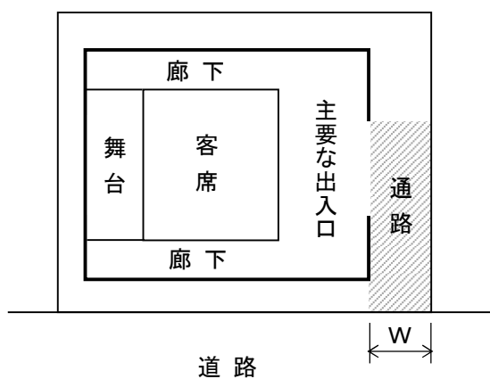
図5-11 出入口が道に面しない場合（第1項）
