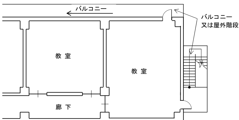
図 5-8 廊下等の出口が 1 箇所でない場合 (第 4 号)
