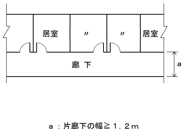
図5-45 片側に居室がある場合
