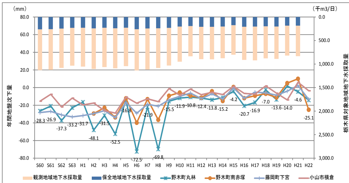
図表3-24 地下水採取量および地盤沈下量の推移（栃木県地盤変動、地下水位調査報告書より作成）
