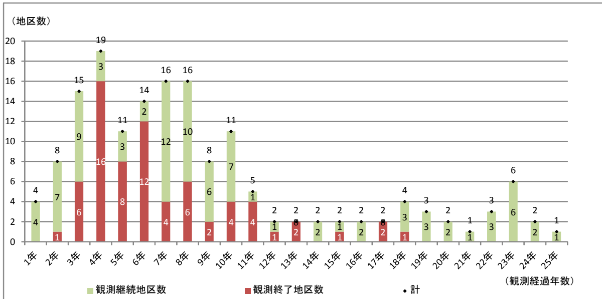
図表3-29 汚染発生からの観測経過年数 (観測継続地区+観測終了地区)
