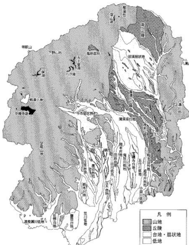
図表3-13 栃木県の地形区分図
