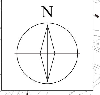
那珂川水系内川洪水浸水想定区域図（家屋倒壊等氾濫想定区域（氾濫流））
