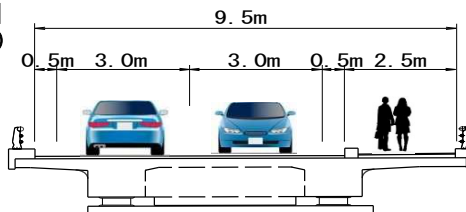
標準横断面図 (留春大橋)
