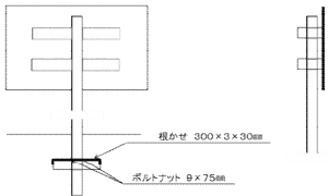
取付構造詳細図
