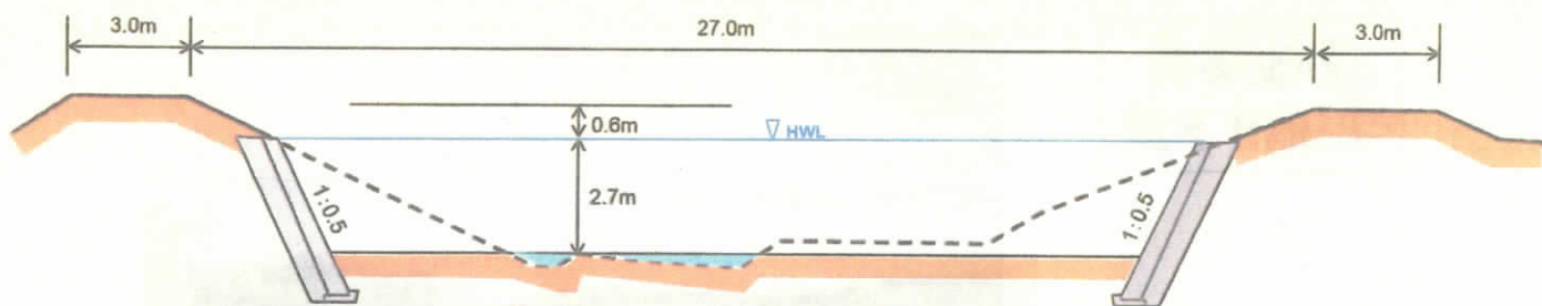
標準断面図
