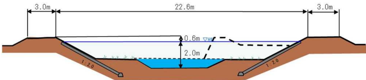
標準断面図
