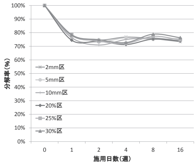
図14 ふるいと水分条件を変えたペレット堆肥の表面施用区における炭素の分解率の変化
