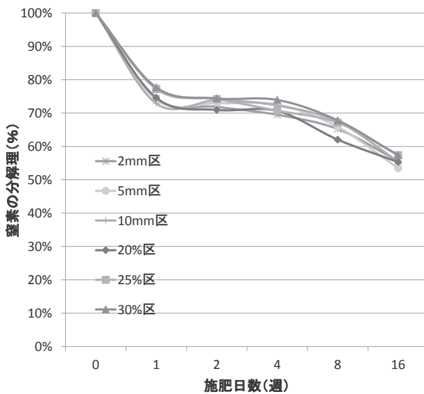
図15 ふるいと水分条件を変えたペレット堆肥の全面施用区における窒素の分解率の変化
