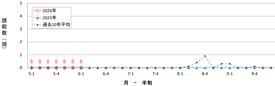
セジロウカの60W予察灯による誘殺数 (栃木市大塚町)
