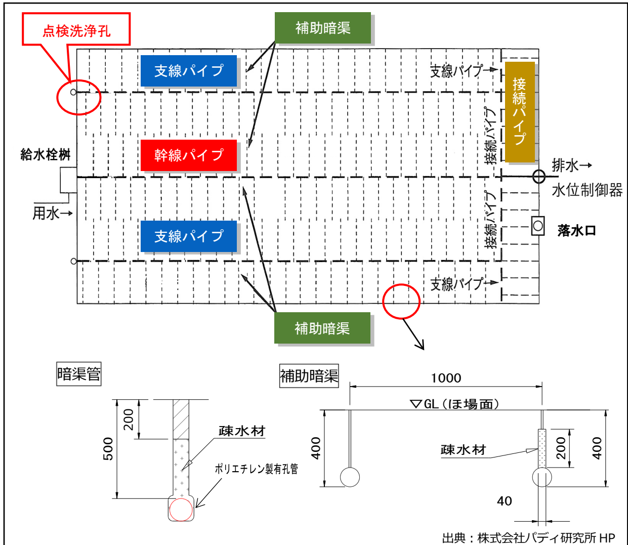
図 5-3-3 FOEAS 概略平面図
