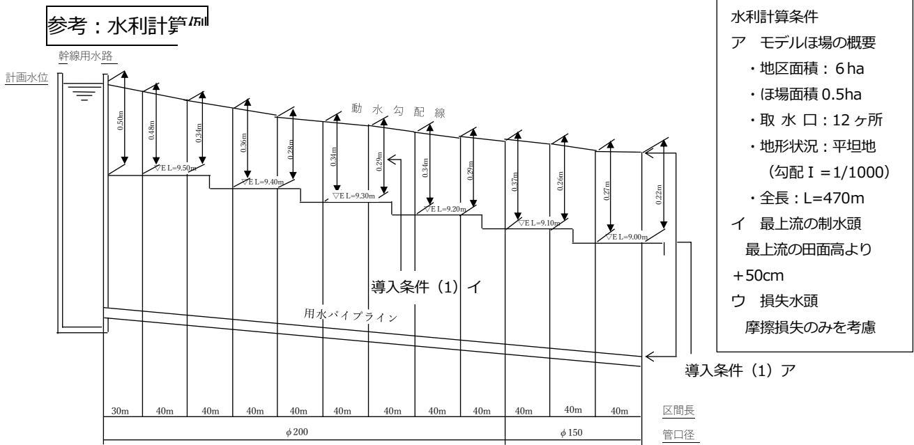
図 5-5-5 水利縦断面図の例
