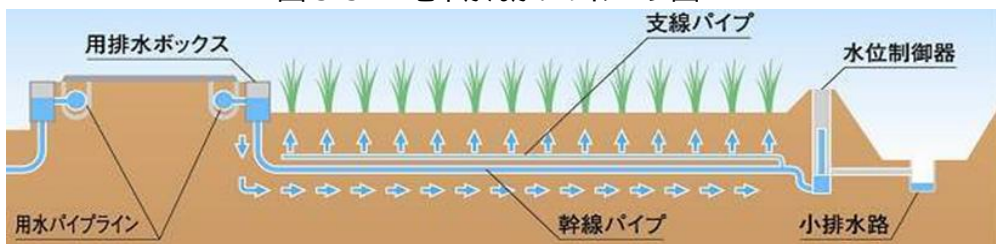
図 5-3-2 地下かんがいのイメージ図
