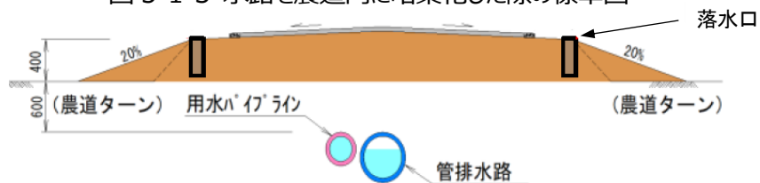
図 5-1-3 水路を農道内に暗渠化した際の標準図
