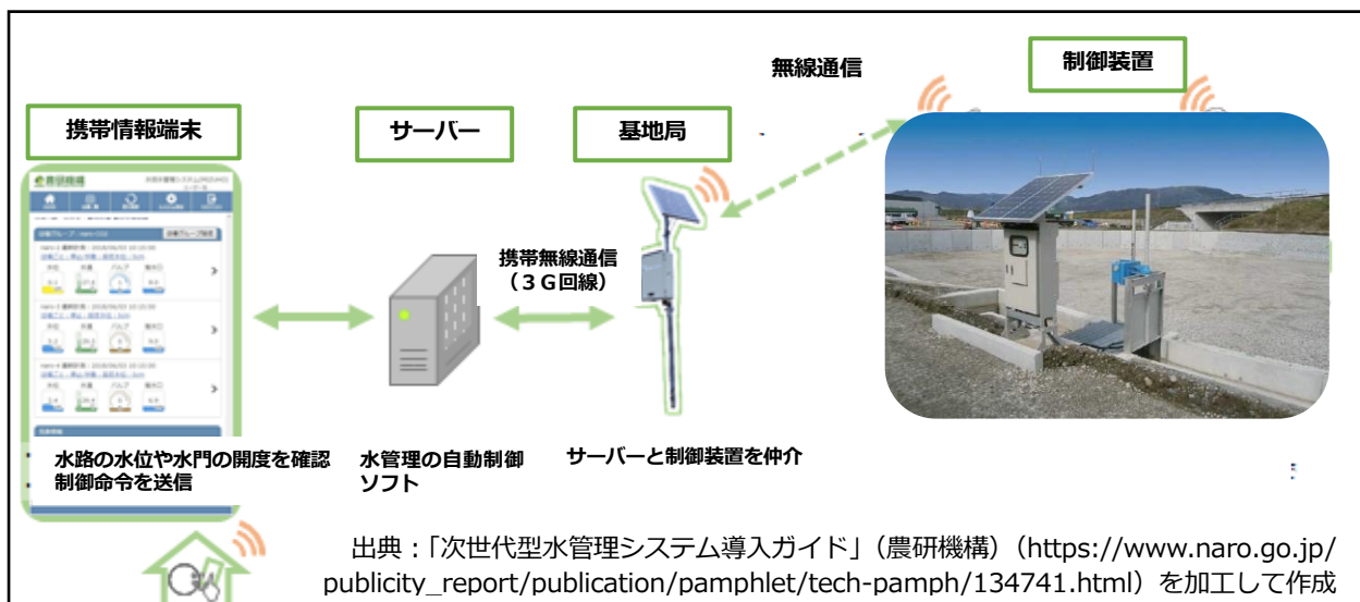
図 5-12-2 水利施設の ICT 化の概要図
