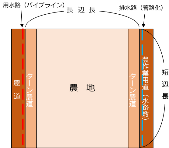
図 5-7-1 ターン農道技術概要図
