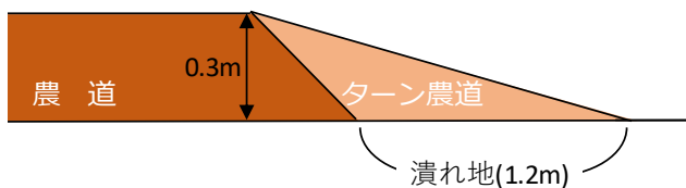
図 5-7-3 ターン農道潰れ地のイメージ
