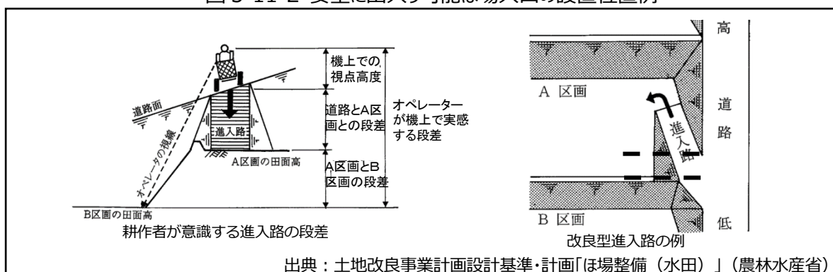
図 5-11-2 安全に出入り可能ほ場入口の設置位置例
