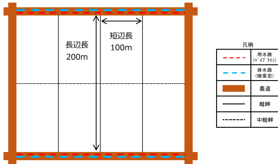
図 5-1-2 長辺長を拡大し更なる大区画化を図る例
