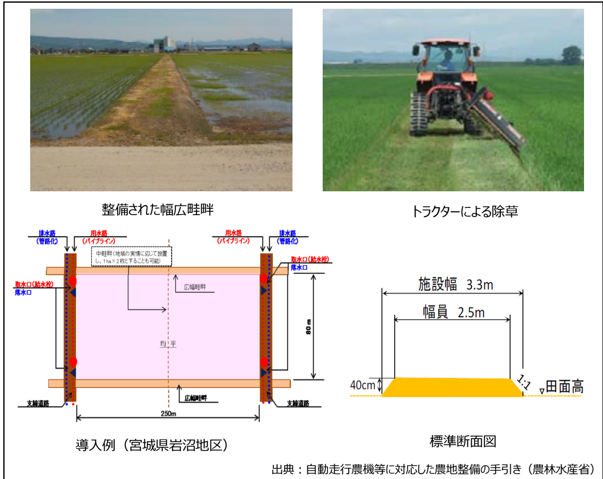
図 5-4-1 幅広畦畔技術概要
