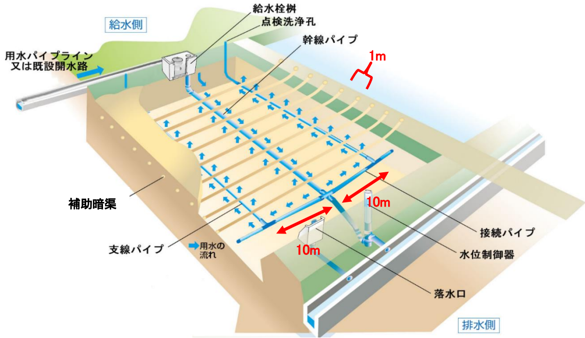
図 5-3-1 FOEAS 模式図
