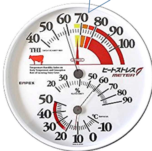
市販のヒートストレスメーター
