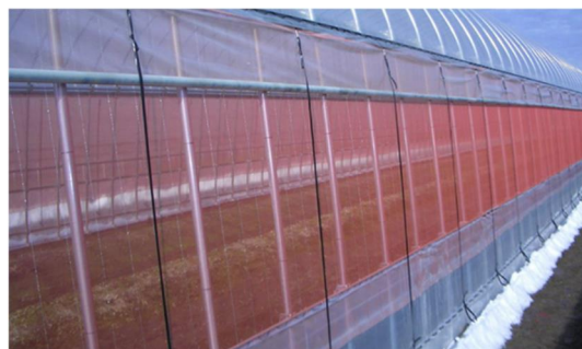
図30 0.4mm目合いの防虫ネット
