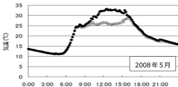
図12 トマトハウスでの細霧冷房による昇温抑止効果 栃木農試 2009 木野本ら（△細霧冷房区、●対照区の温度）
