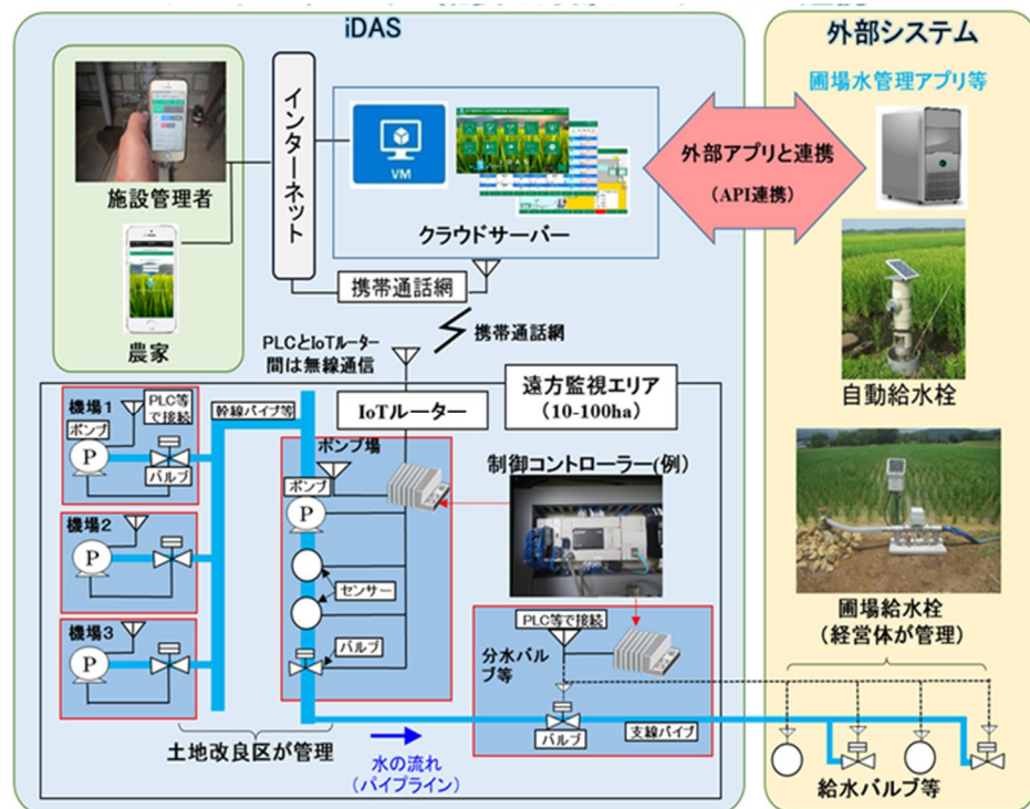
図 20 システム(iDAS)の概要と外部システムとの連携
