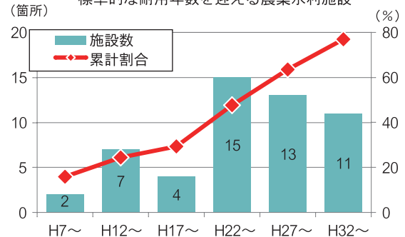
標準的な耐用年数を迎える農業水利施設
