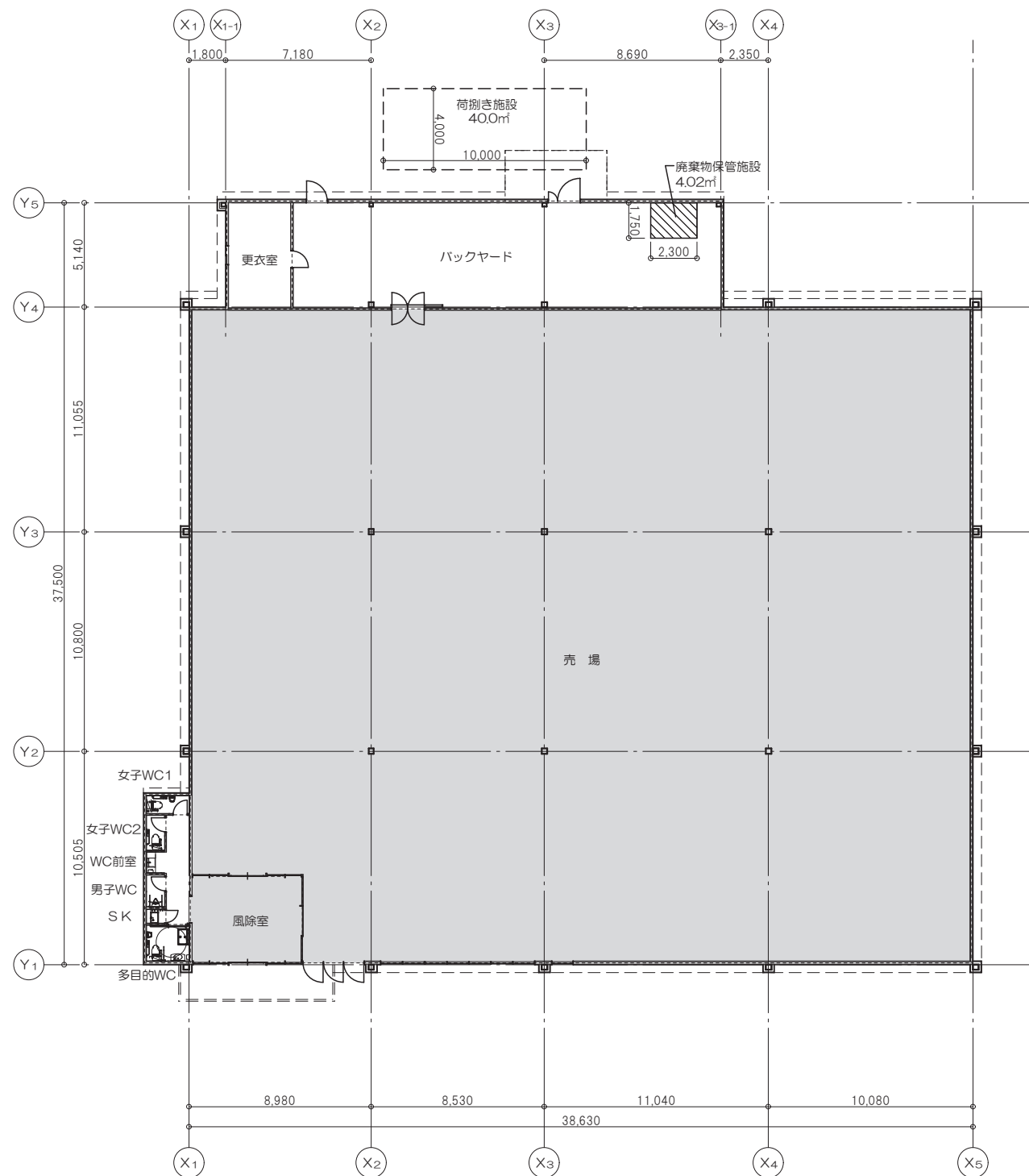
平面図
