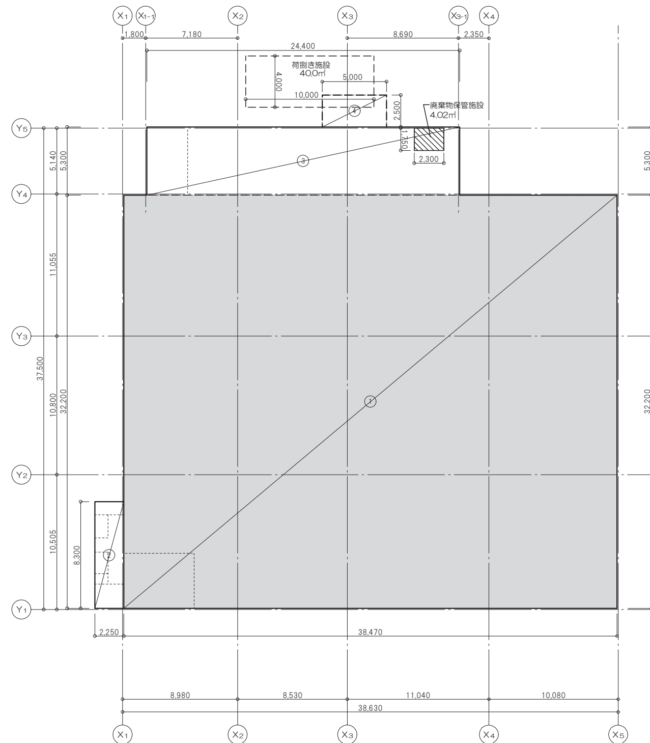
求積図
