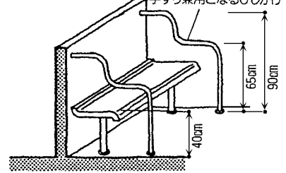
杖使用者用ベンチの例
