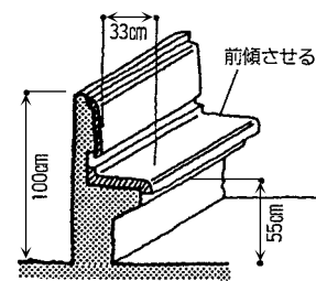
杖使用者用ベンチの例
