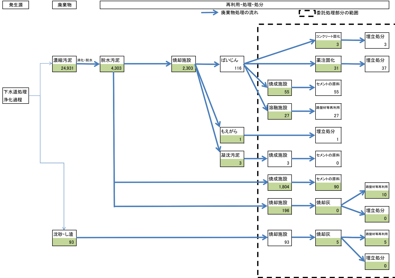
廃棄物処理フロー図(現状)
