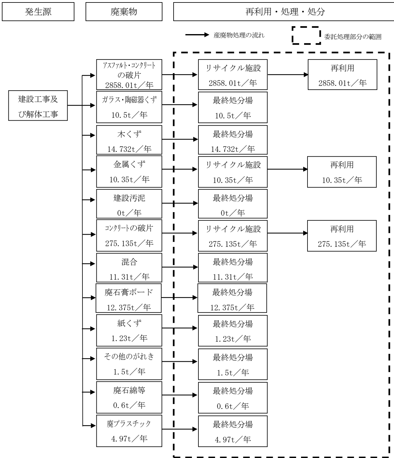
廃棄物処理フロー図（現状）
