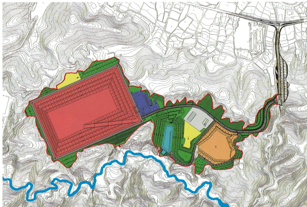
〈配置図〉
