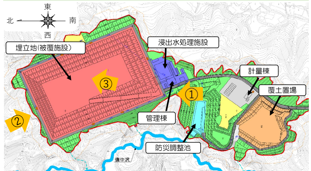
施設配置図
