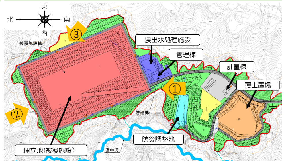
施設配置図
