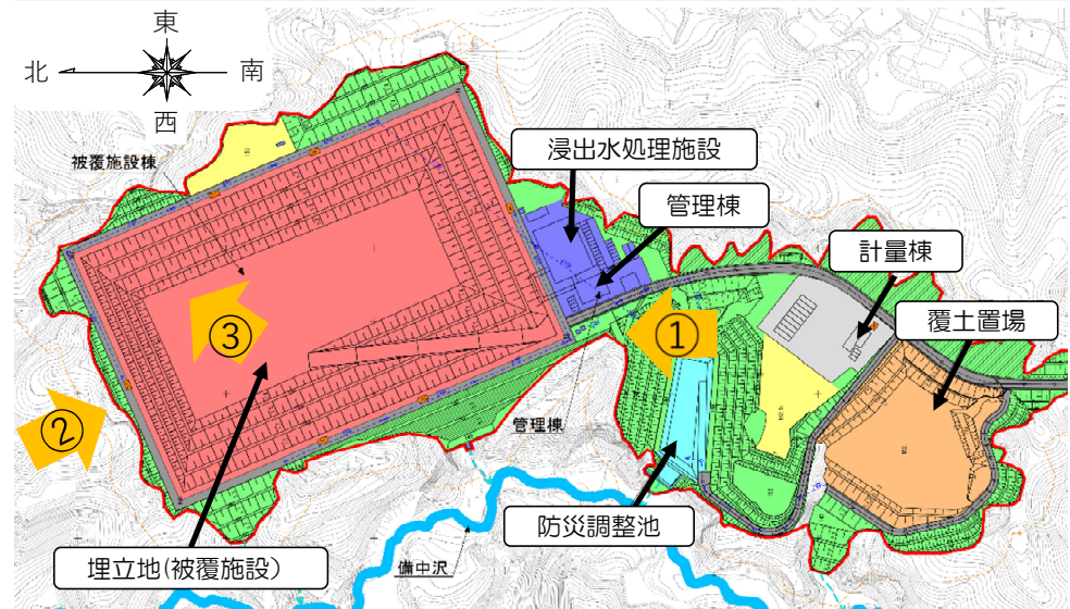
施設配置図
