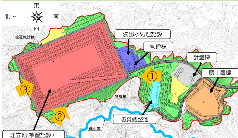
施設配置図
