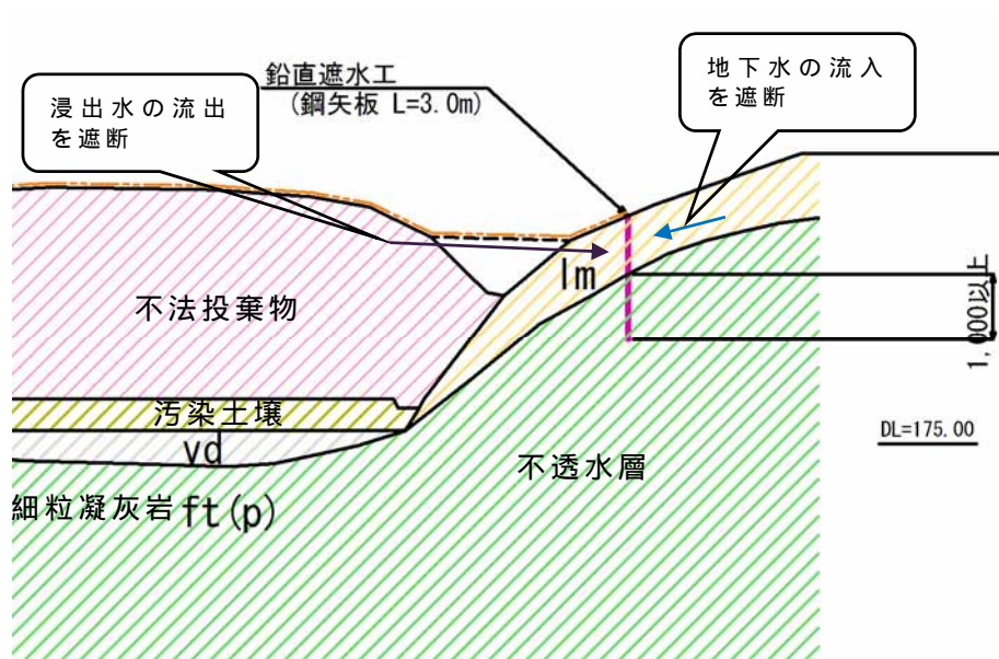
図 4-2-1 鉛直遮水工断面図
