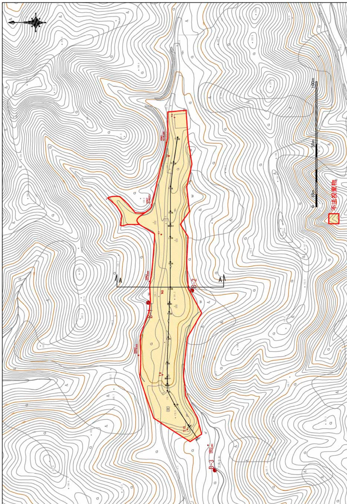
图 2-1-1 現況平面図
