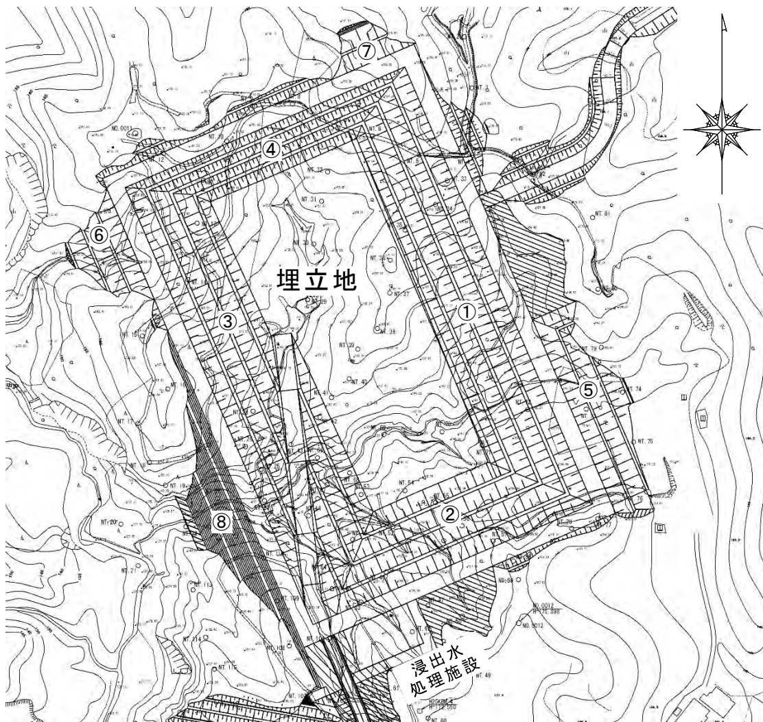
図 4-3-1 埋立地平面図
