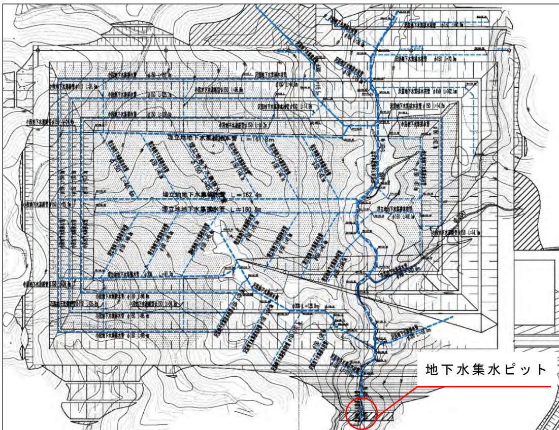
図 4-8-1 地下水集排水施設計画平面図
