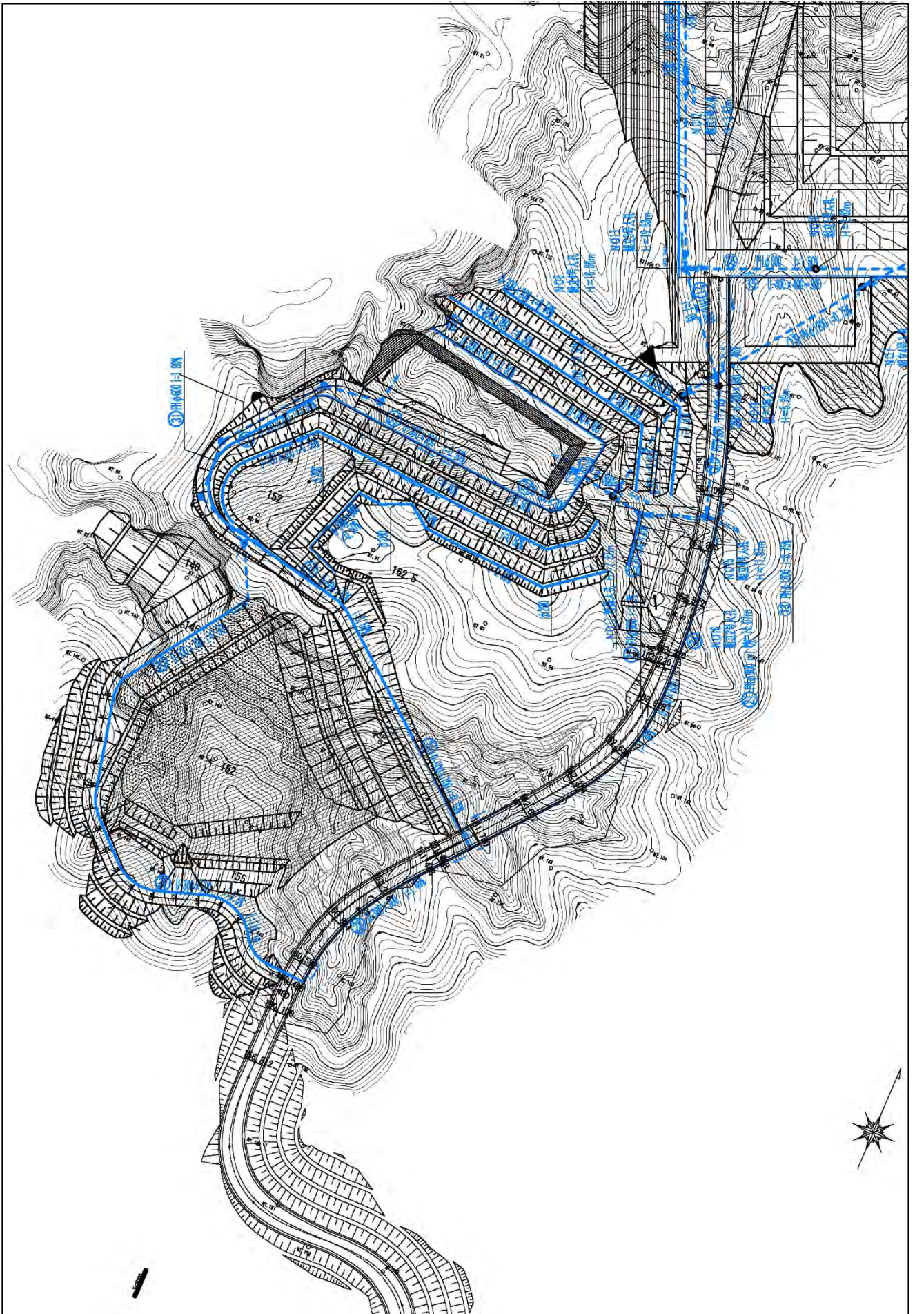
图 4-9-2 雨水集排水施設設計画平面図(2)
