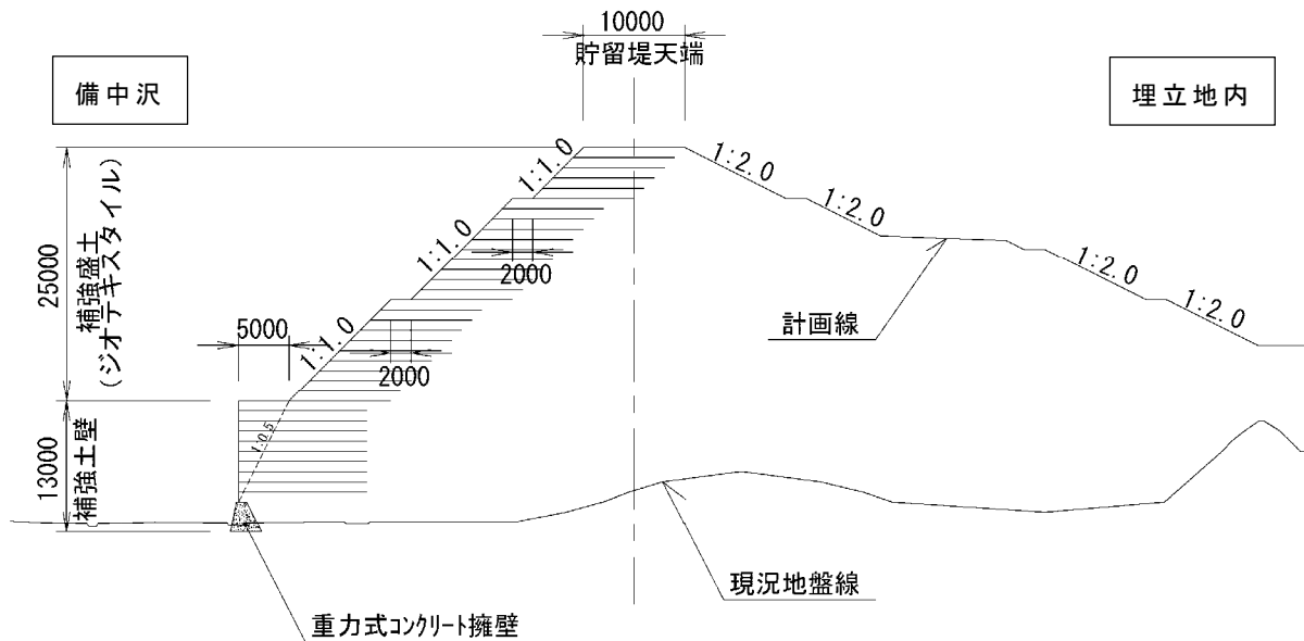
図4-3-4 補強土壁、補強盛土（ジオテキスタイル）の概念図
