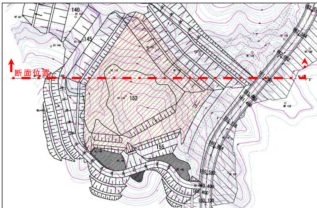
図 4-16-1 覆土仮置場平面図
