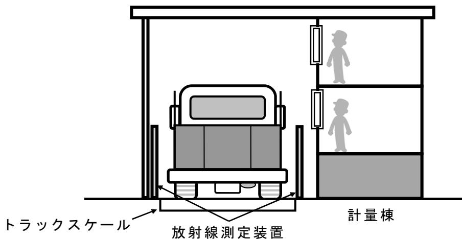
図 4-15-3 搬入管理の概念図
