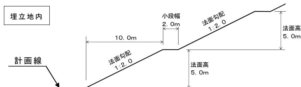
図 4-3-2 法面形状（埋立地東側・南側・西側）
