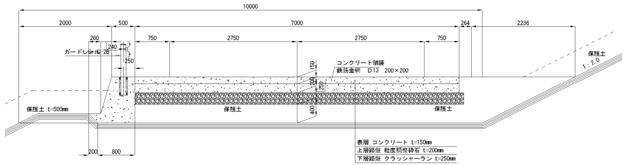
図 4-13-2 場内道路標準断面図
