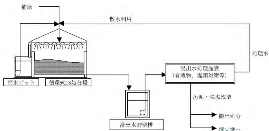
図 4-6-1 循環式概念図
