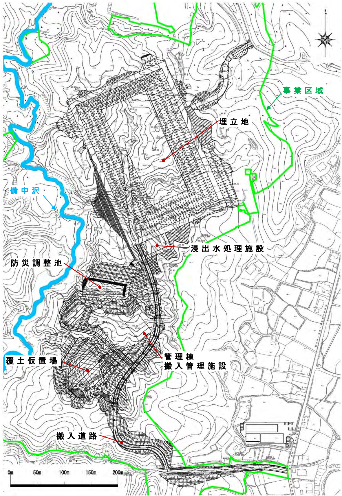
图 4-1 計画平面図
