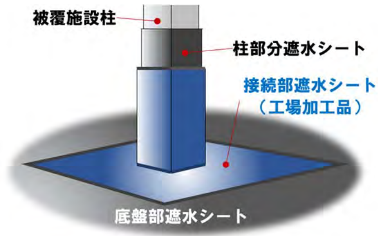
図 4-5-7 被覆施設中間柱底盤部遮水シート概念図
