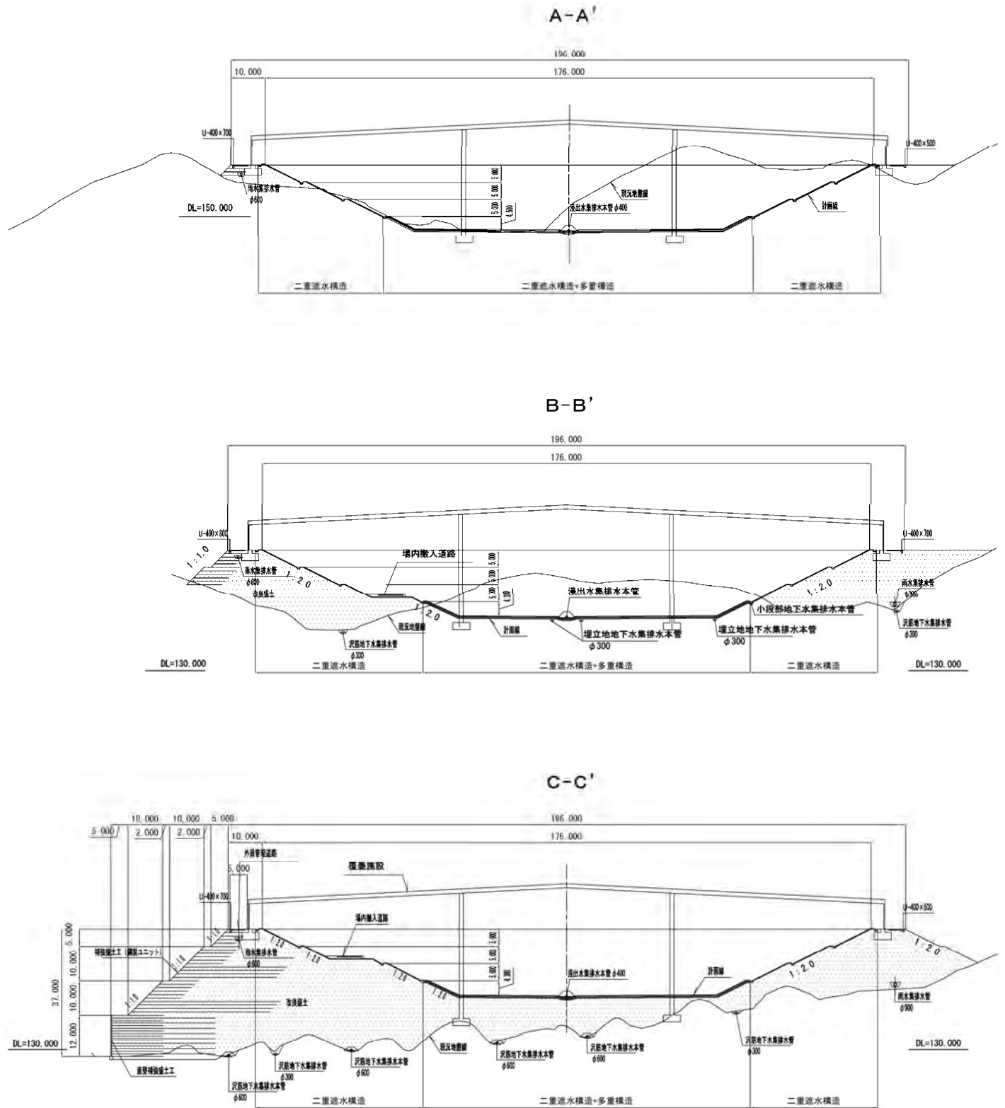
图 4-2-2 代表横断面图
