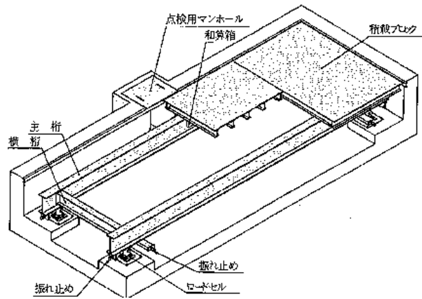
図 4-15-2 計量施設の概念図
