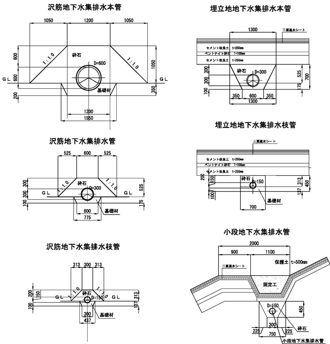
図 4-8-2 地下水集排水管構造図
