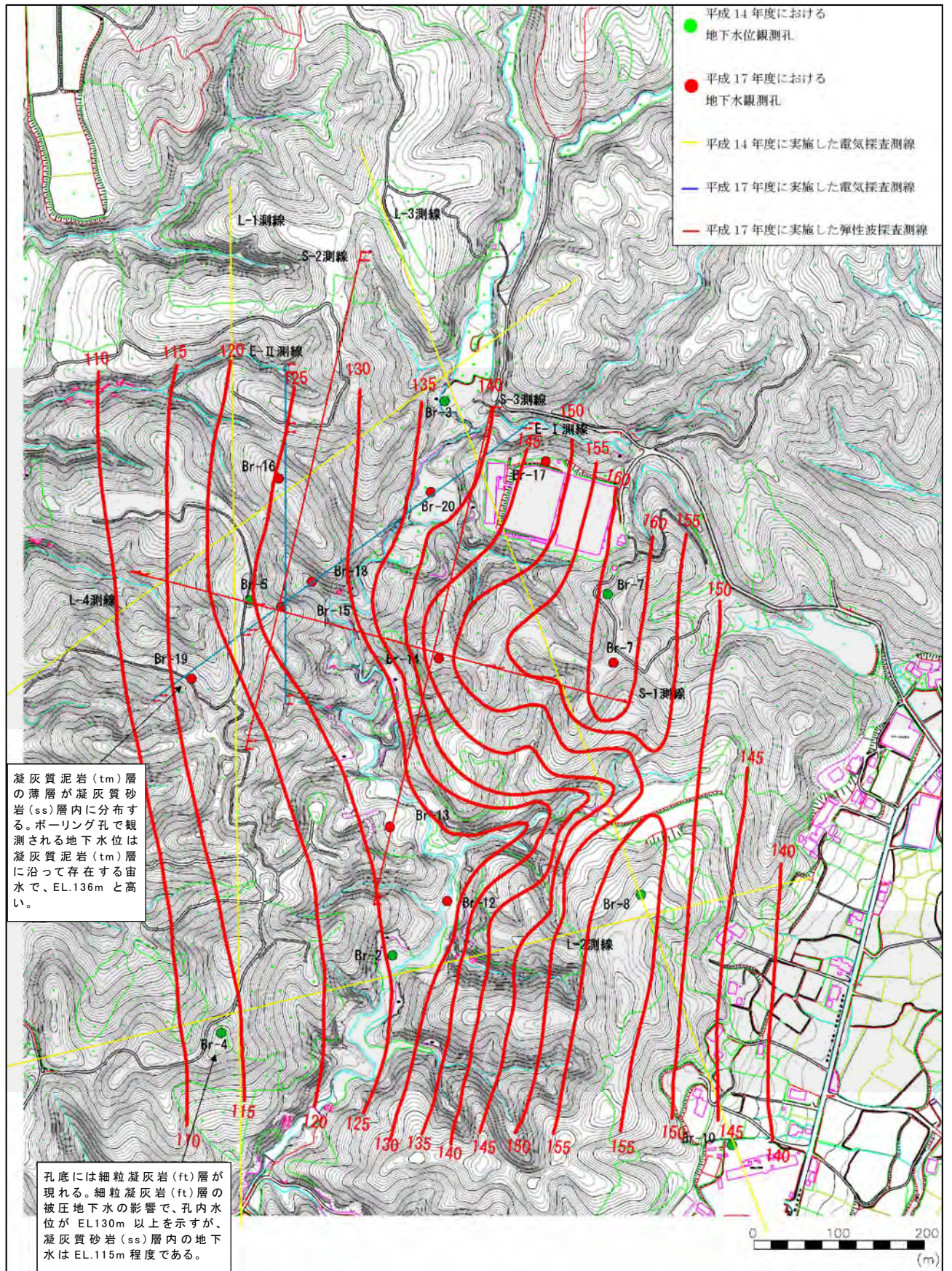
図 2-3-2 凝灰質砂岩 (ss) 層の地下水位分布
