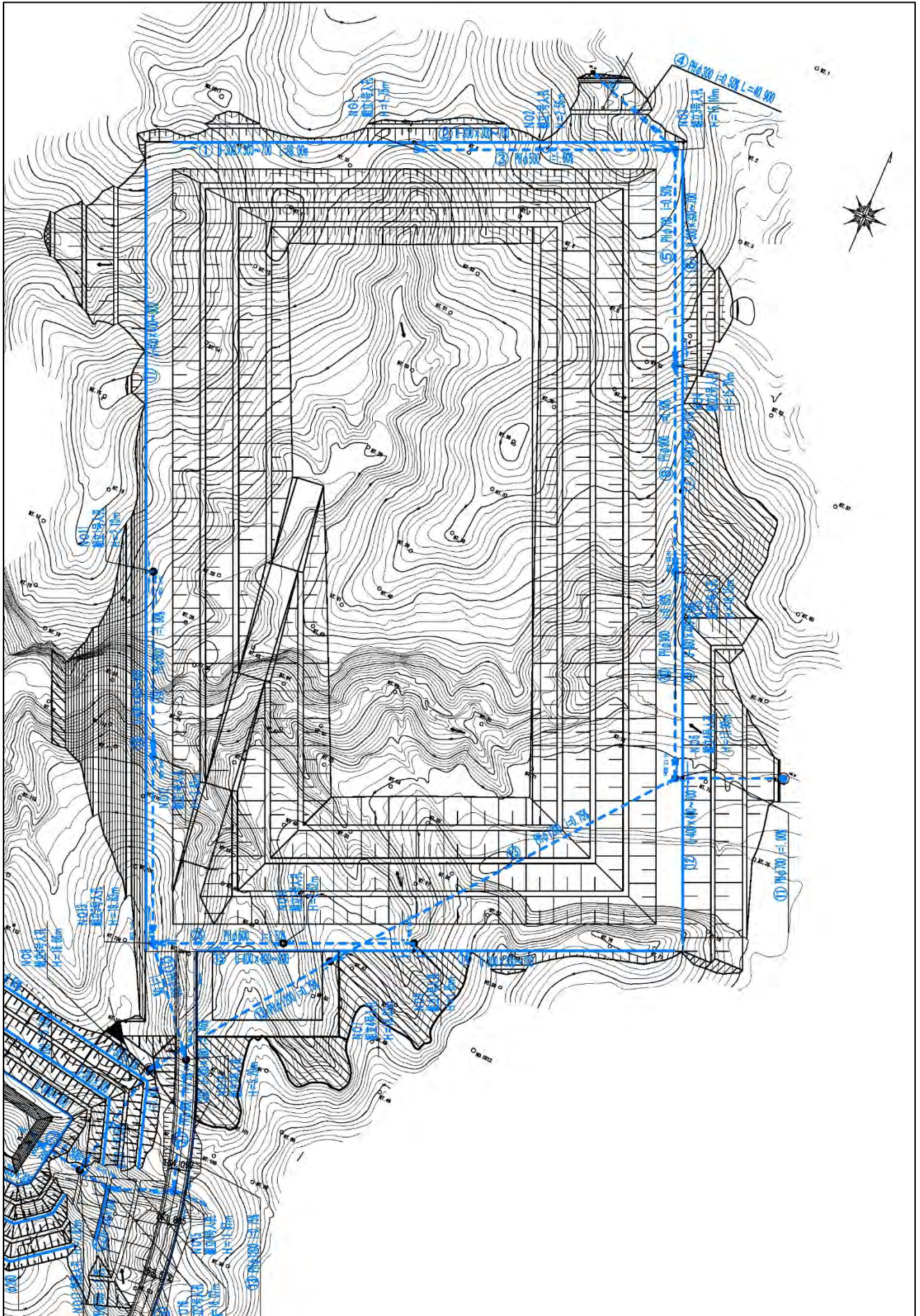
图 4-9-1 雨水集排水施设计画平面图(1)
