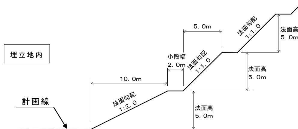
図 4-3-3 法面形状（埋立地北側）
