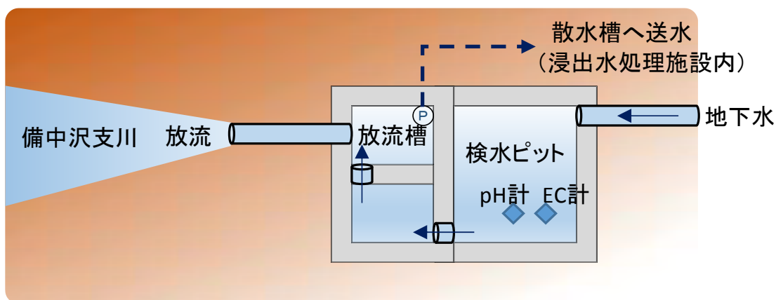
図 4-8-4 地下水集水ピット概念図（平面図）
