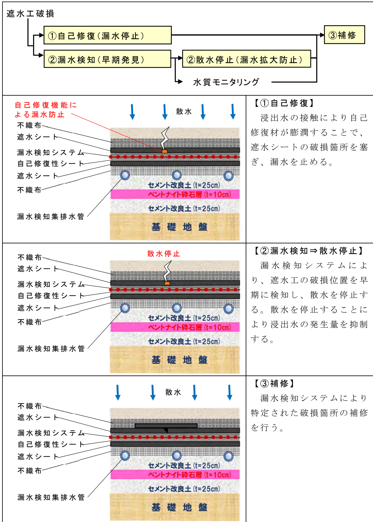
図 4-5-3 漏水対策
