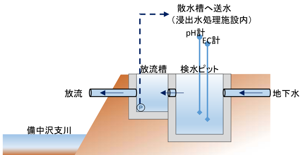
図 4-8-3 地下水集水ピット概念図（断面図）
