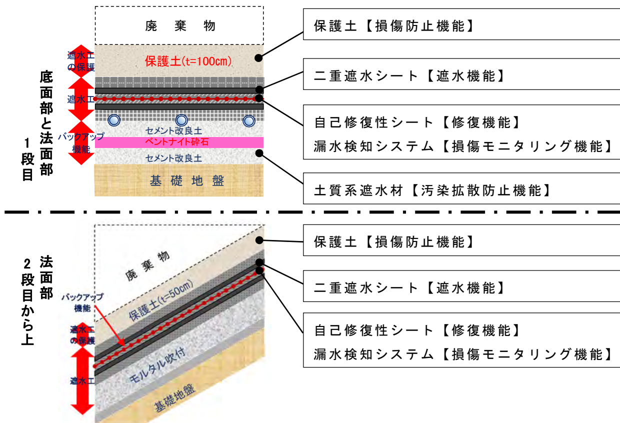
図 4-5-1 二重遮水シートを基本とした多重の遮水構造の模式図
