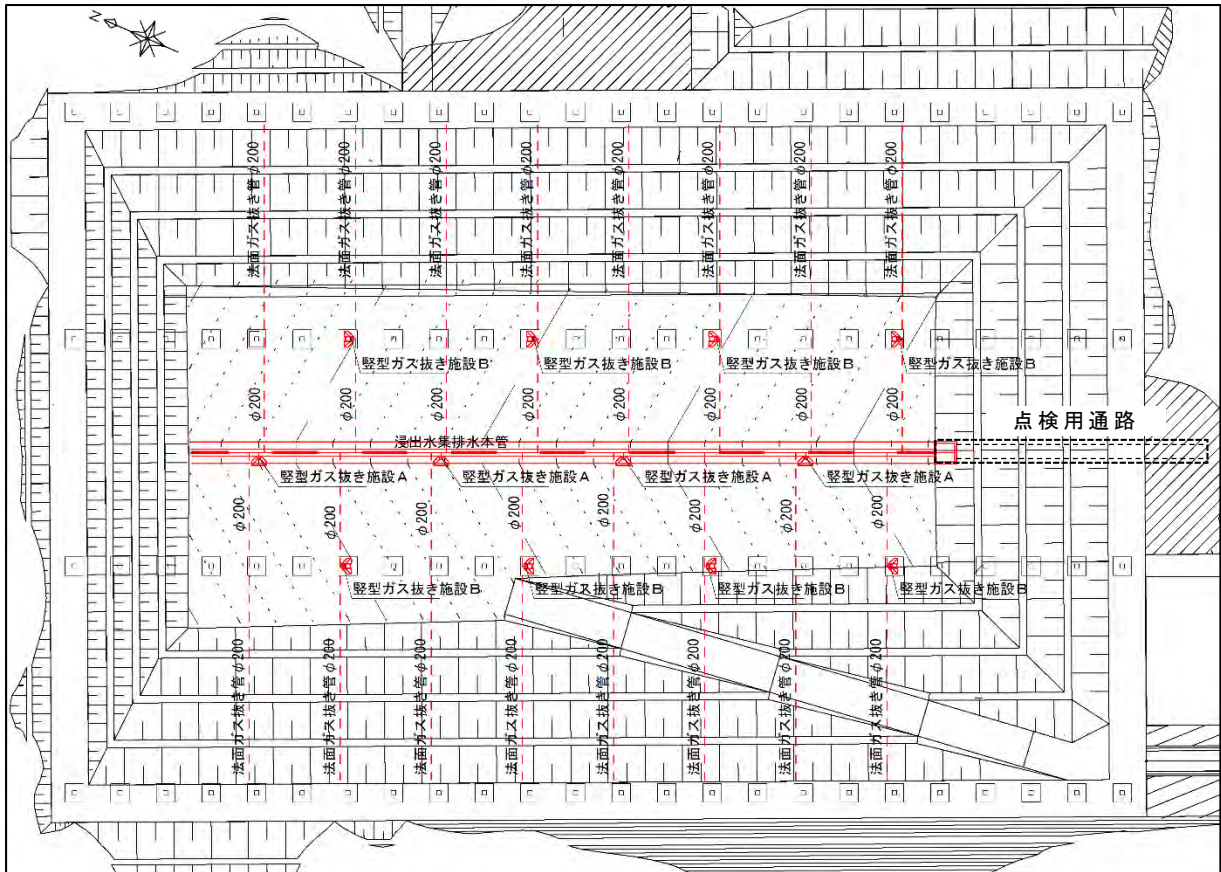
図 4-10-1 埋立ガス抜き施設計画平面図
