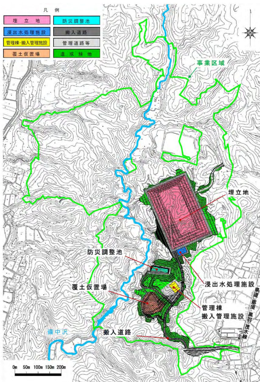
図 3-4 施設配置図
