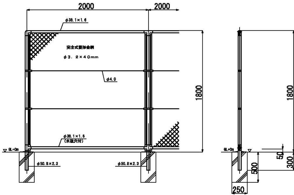
図 4-14-2 フェンス構造図
