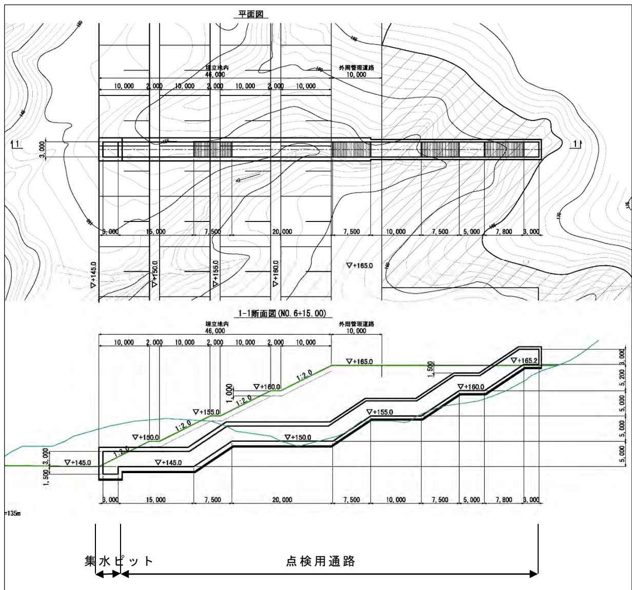
図 4-7-4 浸出水集水ピット計画図
