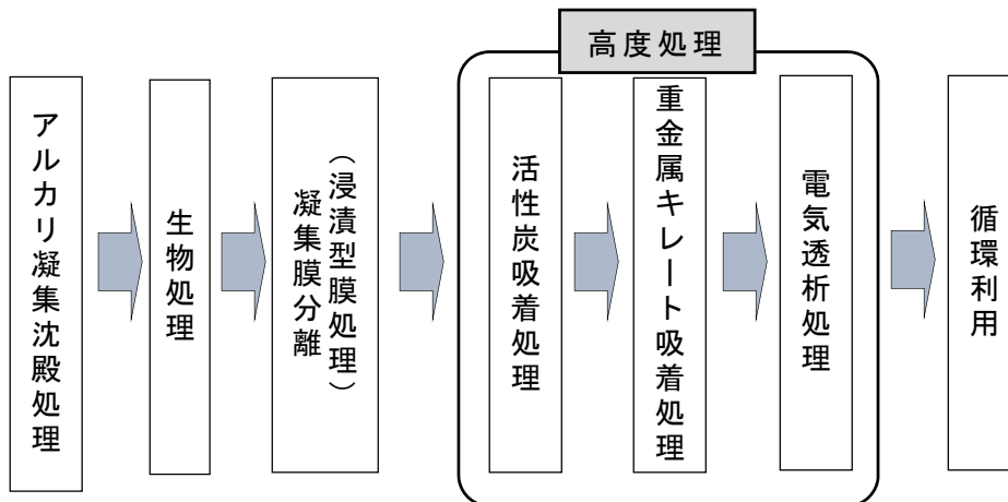
図 4-6-3 浸出水処理フロー
