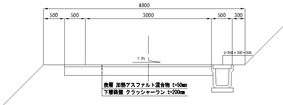
図 4-13-4 管理道路標準断面図
