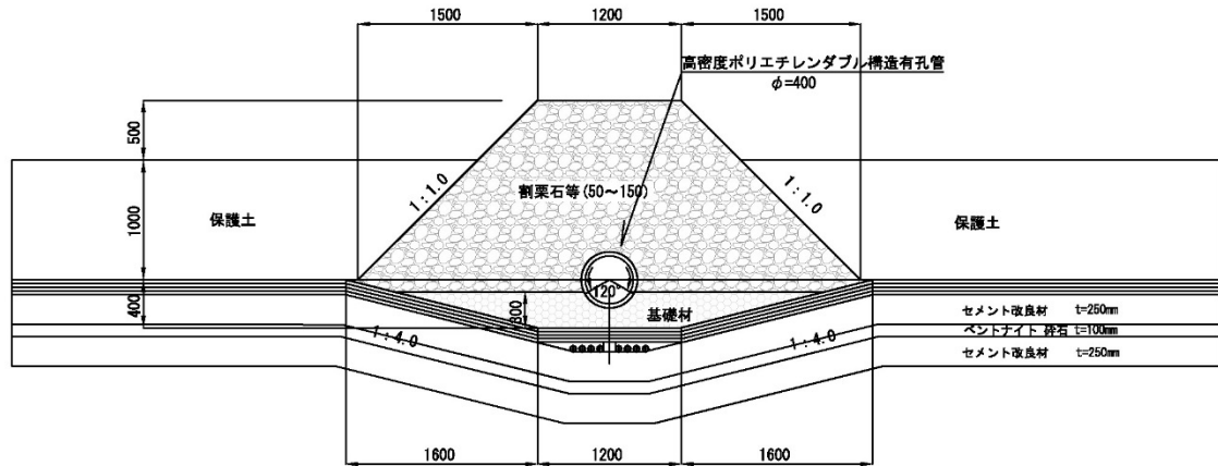
図 4-7-2 浸出水集排水本管構造図
