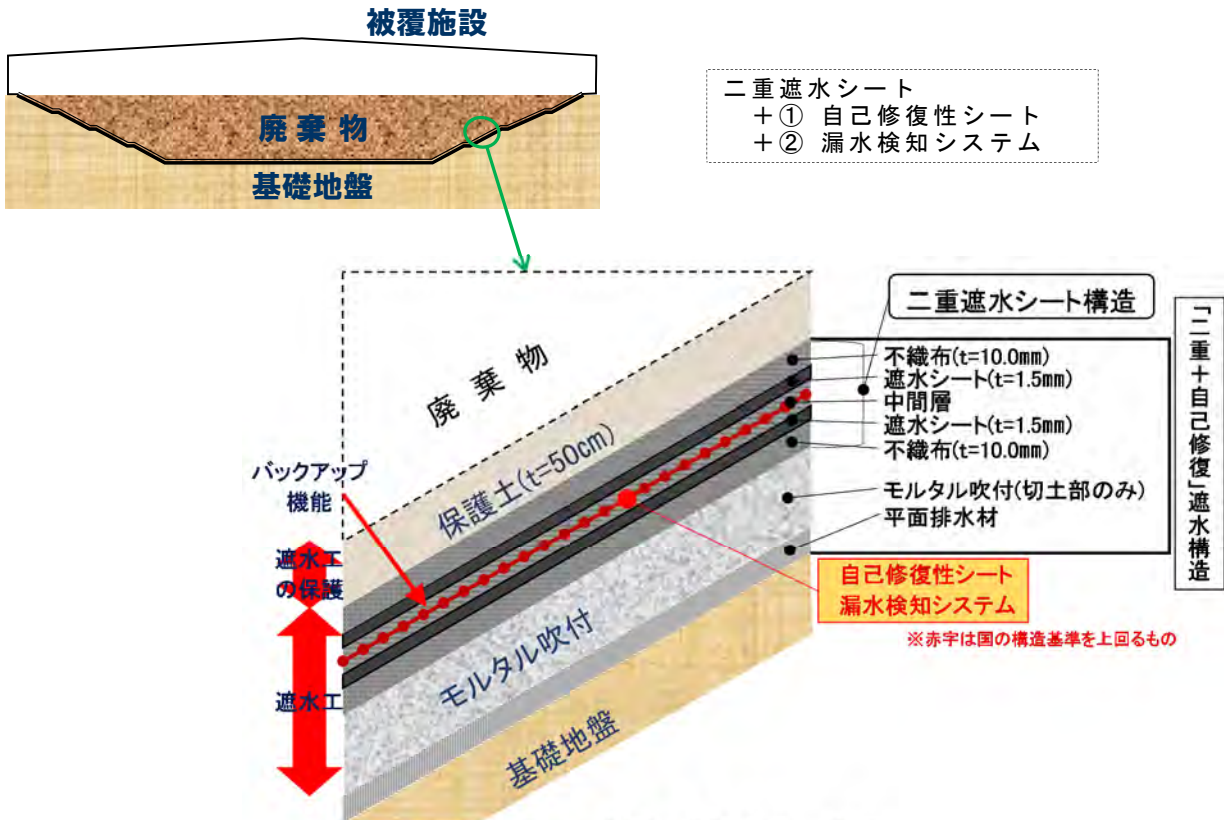
図 4-5-4 遮水構造イメージ図
