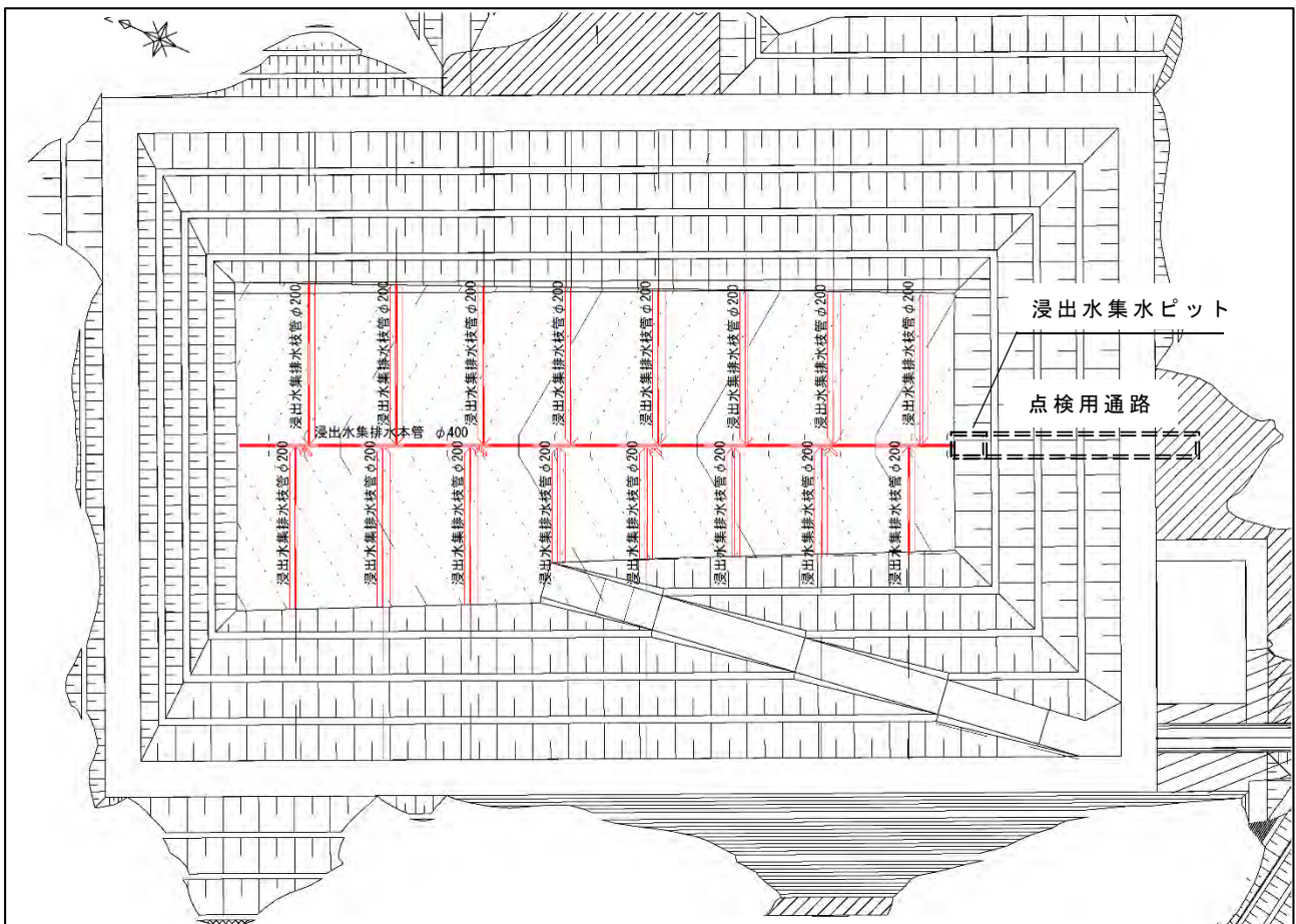
図 4-7-1 浸出水集排水施設計画平面図
