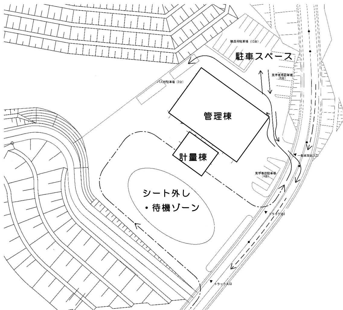
図 4-15-1 管理施設等配置計画
