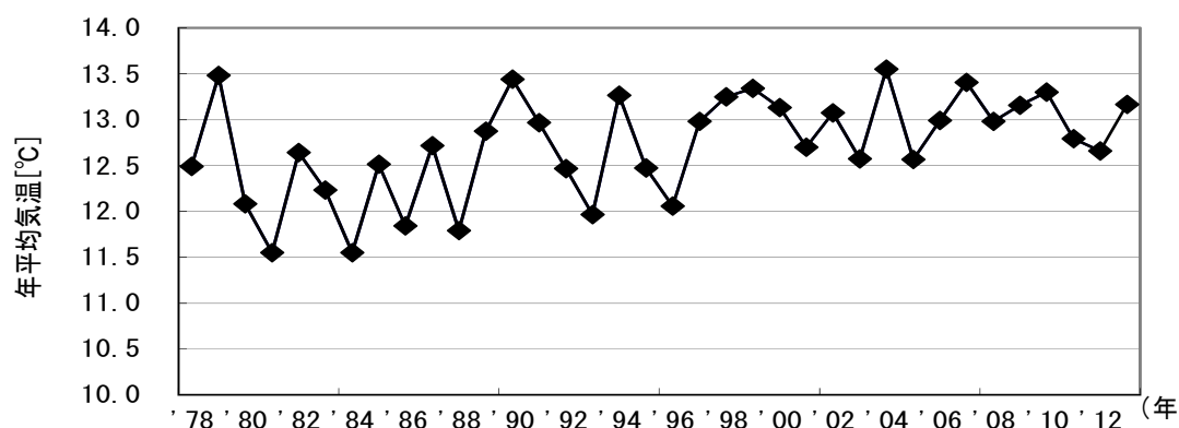
図 2-4 年平均気温の年次変化
