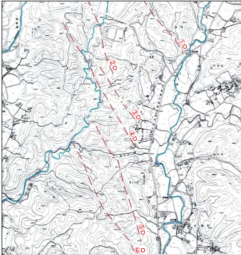
図 2-3-1 リニアメント判読結果
