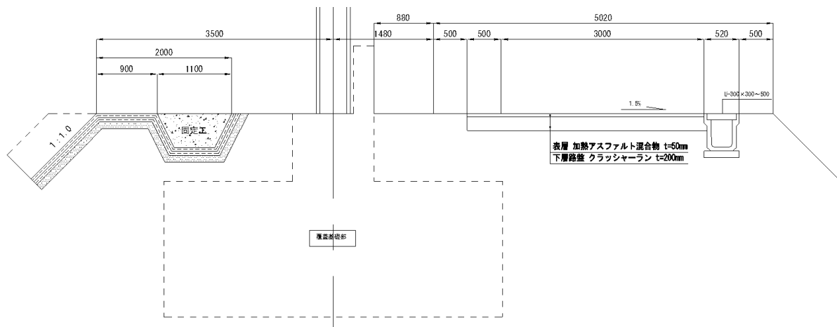
図 4-13-5 管理道路(埋立地外周)道路標準断面図
