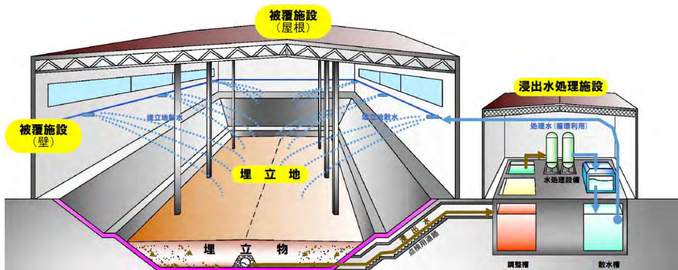
図 3-5 クローズド型最終処分場の概念図
