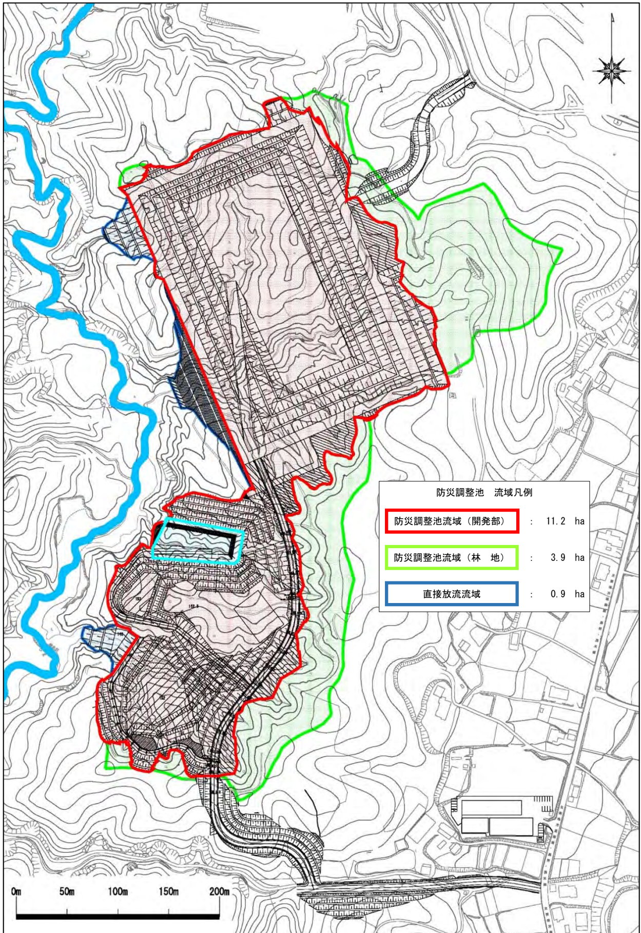
图 4-12-2 防災調整池平面图
