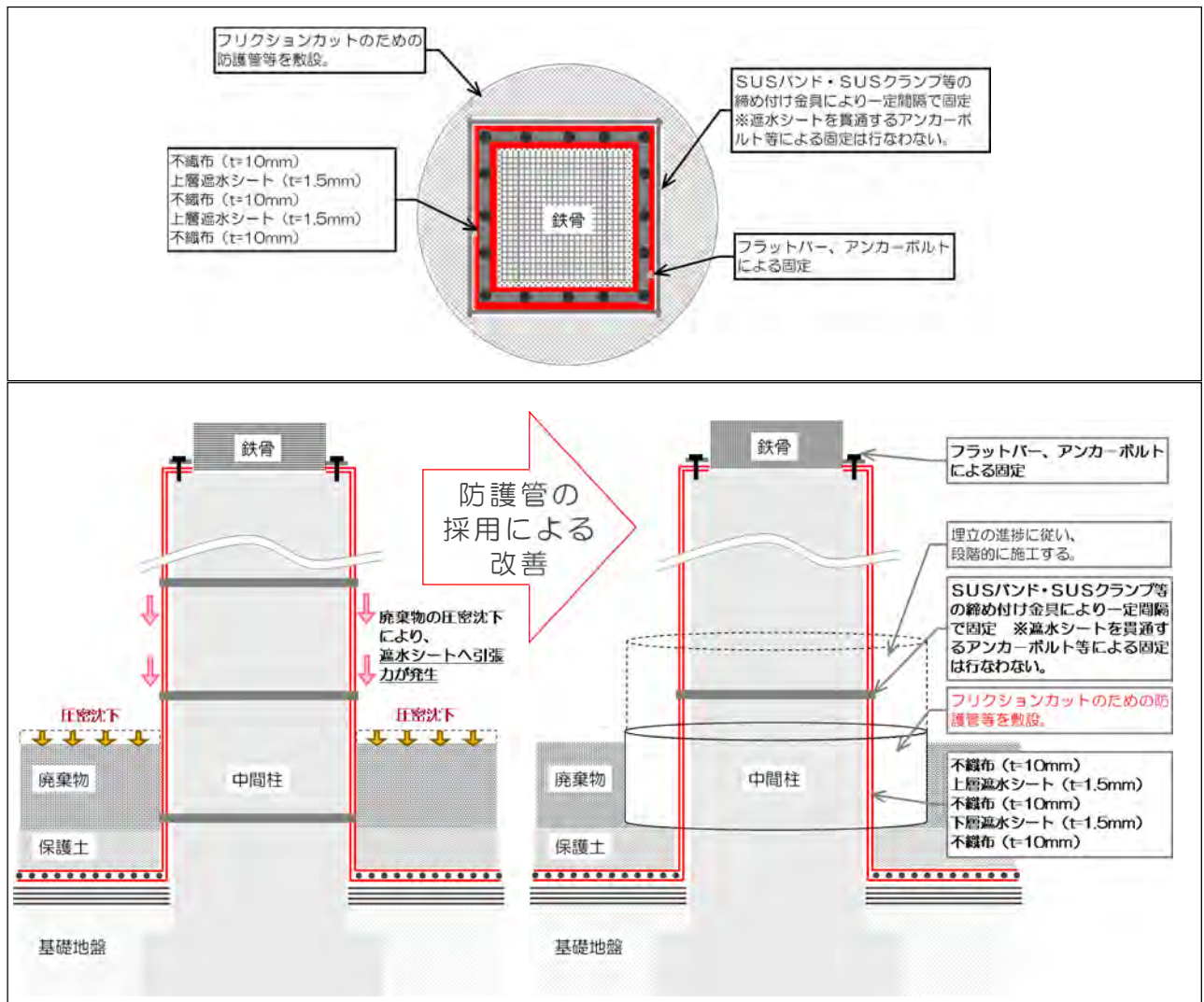
図 4-5-6 被覆施設中間柱構造：上面図(上)・正面図(下)
