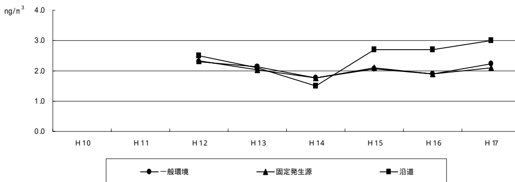
水銀濃度の推移〔年平均値〕
