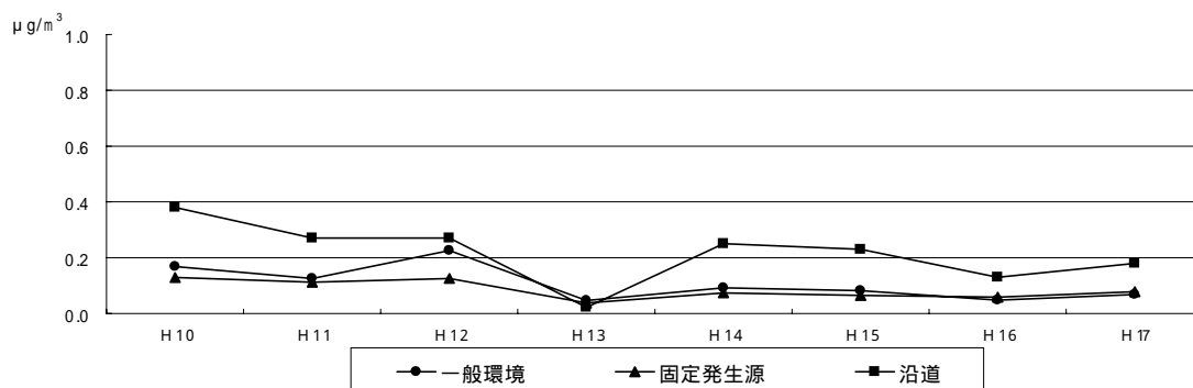
アクリロニトリル濃度の推移〔年平均値〕
