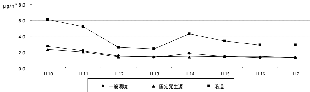
ベンゼン濃度の推移〔年平均値〕
