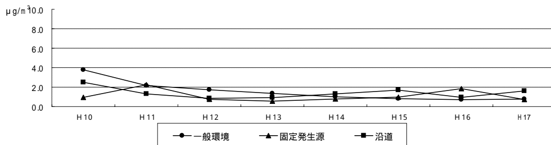
トリクロロエチレン濃度の推移〔年平均値〕
