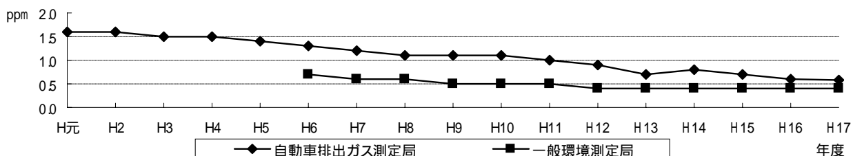
一酸化炭素濃度の推移〔一般局及び自排局 年平均値〕
