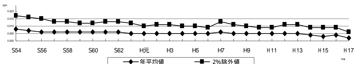
二酸化硫黄濃度の推移〔年平均値・2%除外値〕
