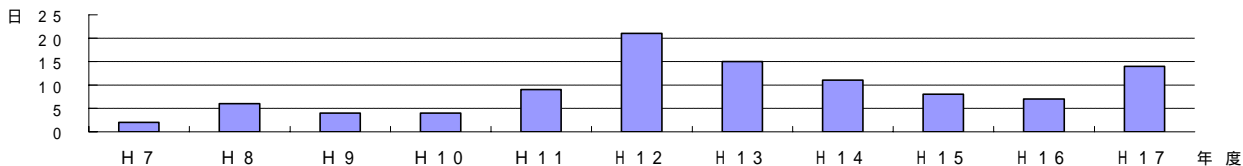
平成17年度 昼間（5～20時）の光化学オキシダント濃度〔月別〕
