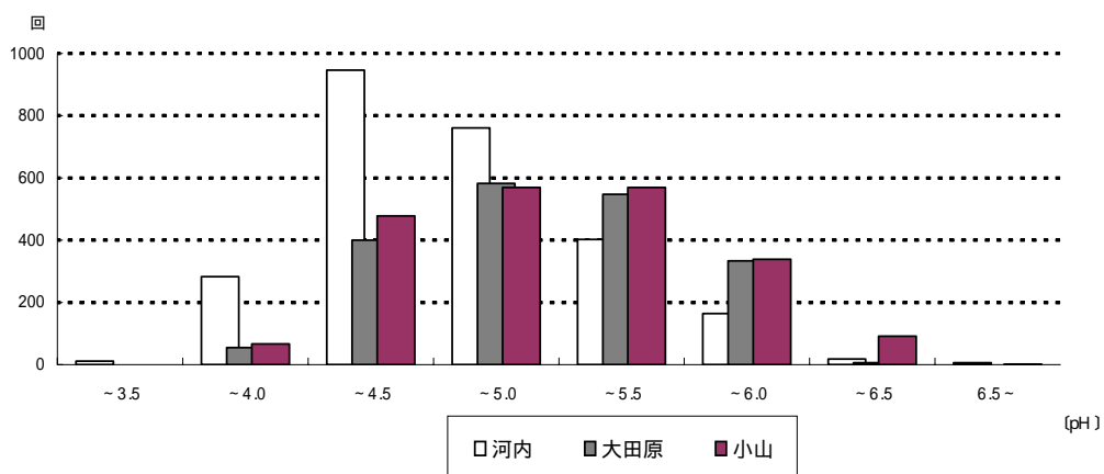
図4-2 調査地点における降水量0.5mmごとのpH頻度分布
