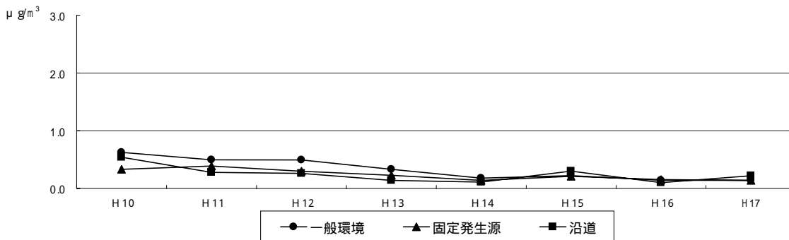
テトラクロロエチレン濃度の推移〔年平均値〕
