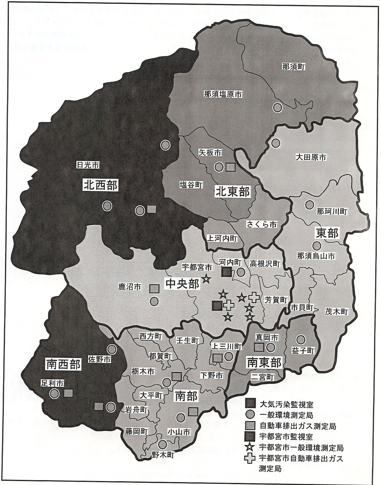
図 2 - 1 大気汚染監視網
