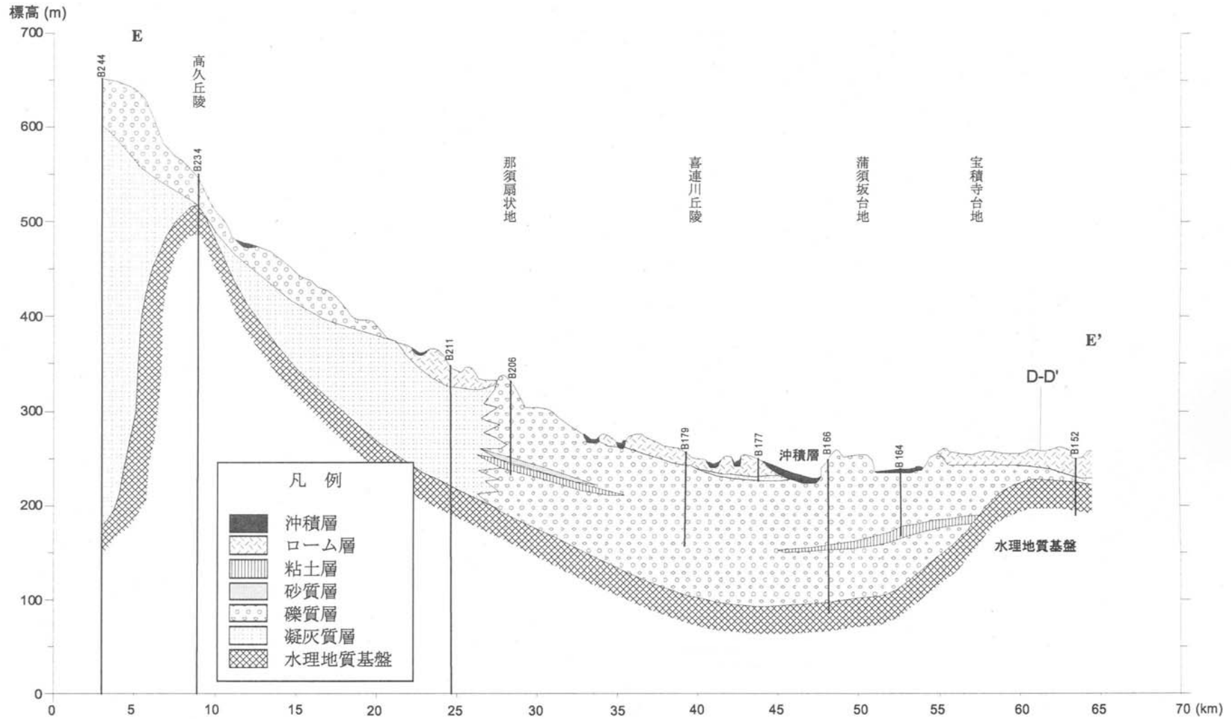
図-16 水理地質断面図 (E-E' 断面)
