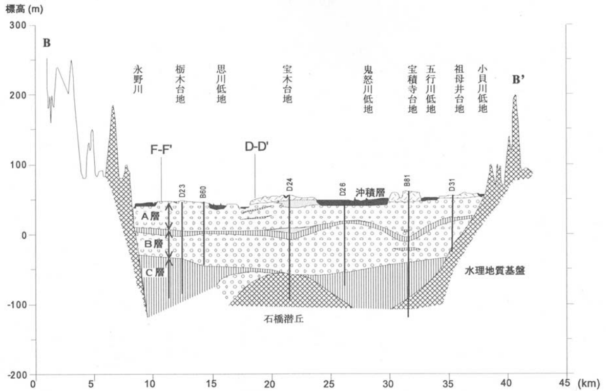
図-14 水理地質断面図 (B-B' 断面、C-C' 断面)
