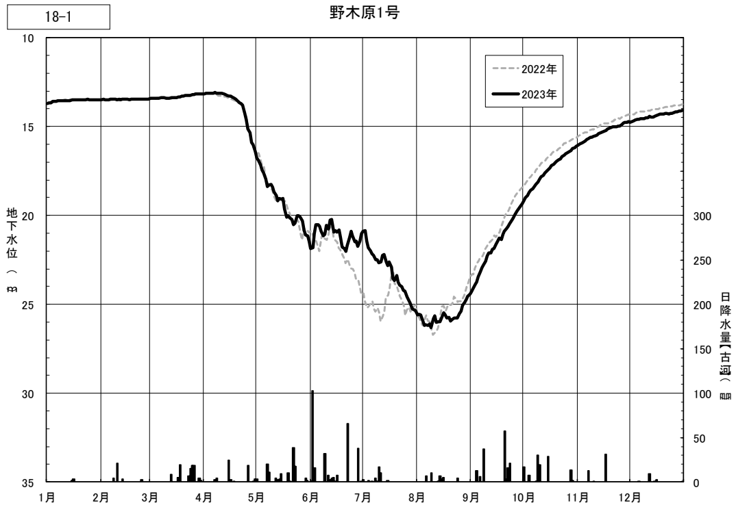
図4.3(43) 日地下水位の年間変動（野木原1号）
