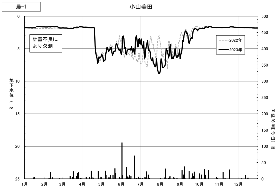
図 4.3(49) 日地下水位の年間変動（小山美田）
