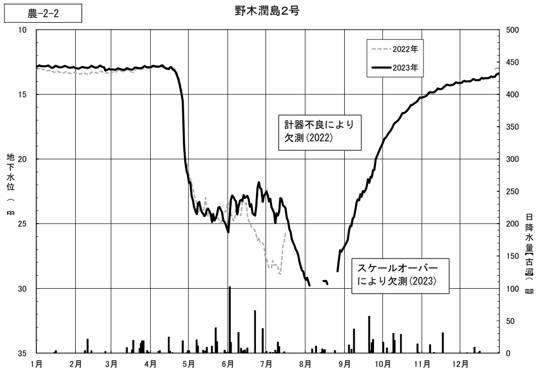
図4.3(53) 日地下水位の年間変動（野木潤島2号）
