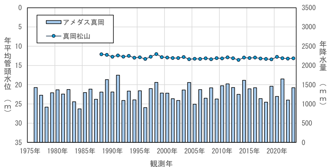
図4.3(73) 年平均地下水位の経年変化（真岡松山）
