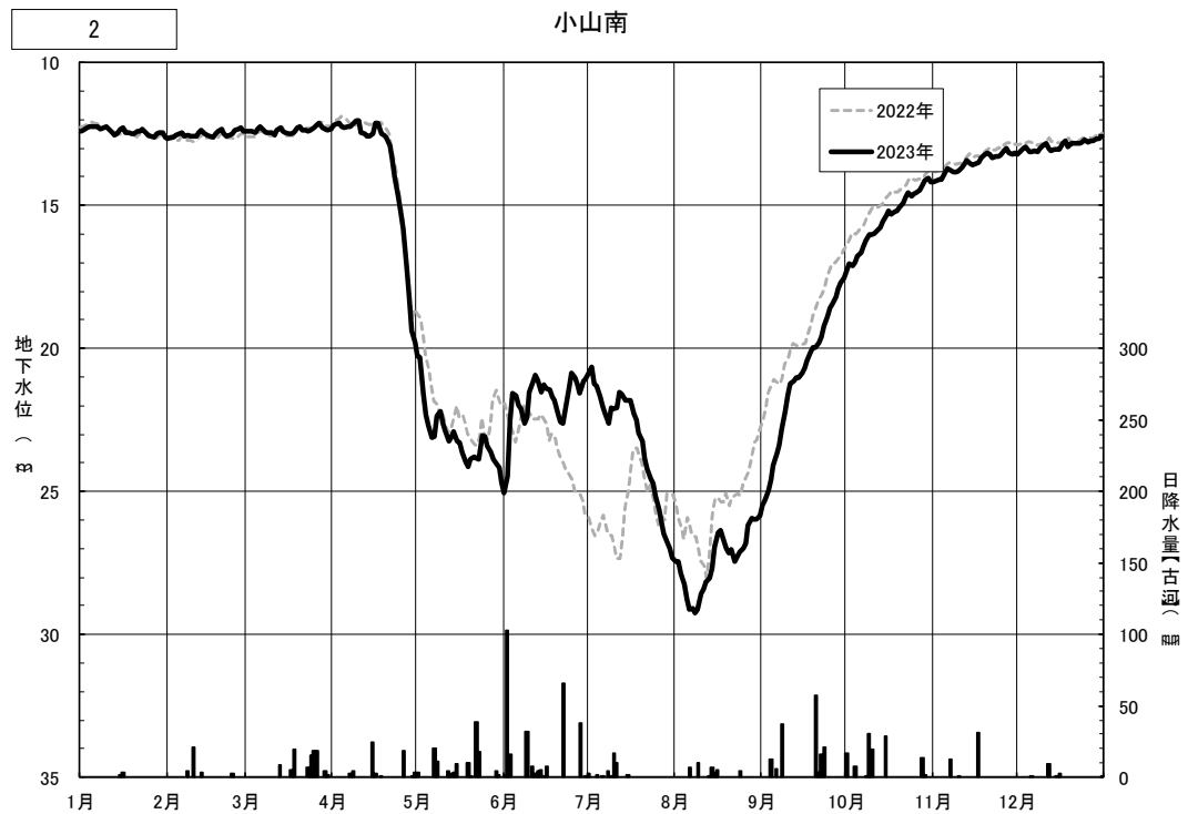
図 4.3(6) 日地下水位の年間変動 (小山南)
