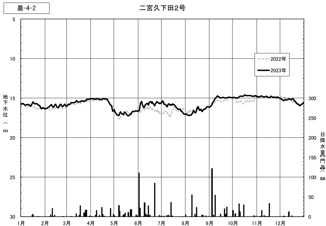
図4.3(89) 日地下水位の年間変動（二宮久下田2号）
