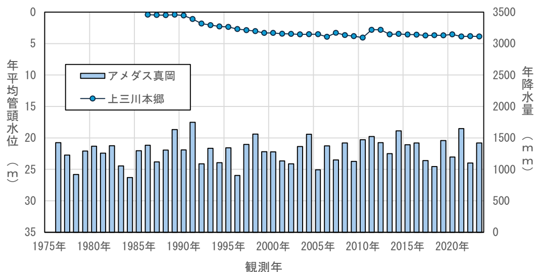
図4.3(81) 年平均地下水位の経年変化（上三川本郷）
