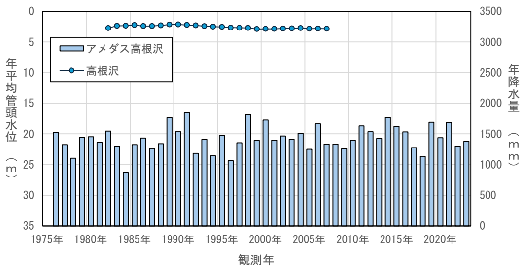
図4.3(96) 年平均地下水位の経年変化（高根沢）
