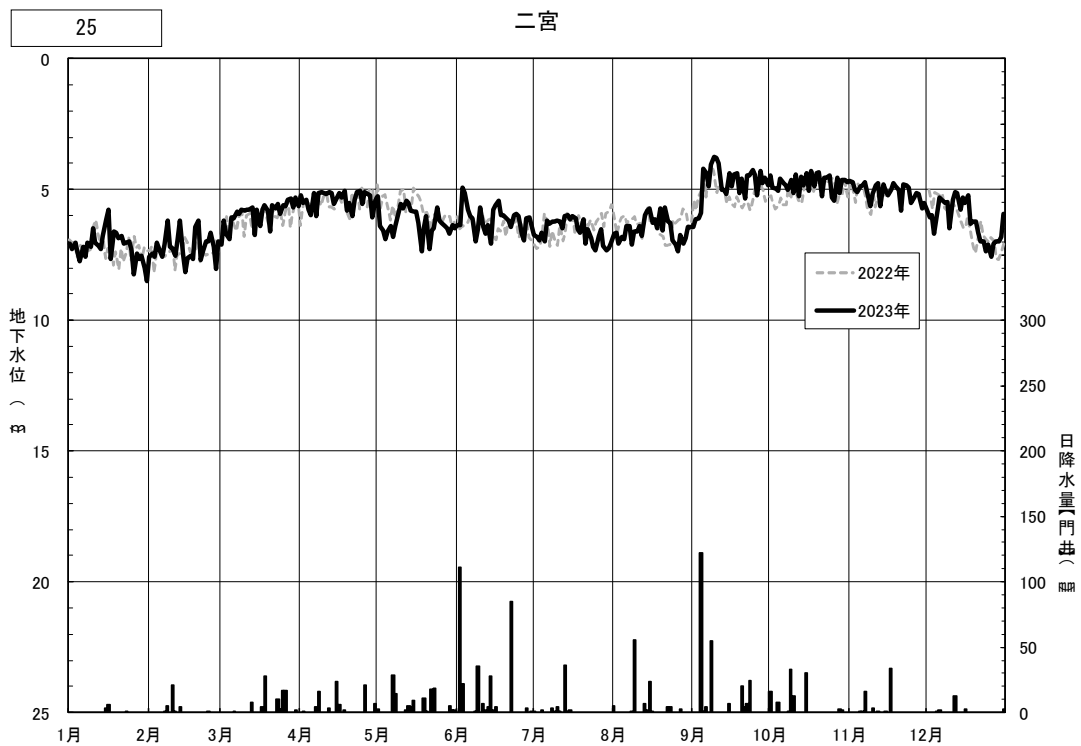
図4.3(76) 日地下水位の年間変動（二宮）
