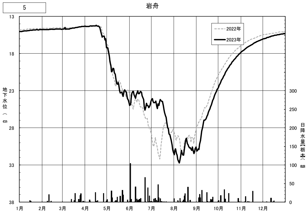
図 4.3(11) 日地下水位の年間変動（岩舟）
