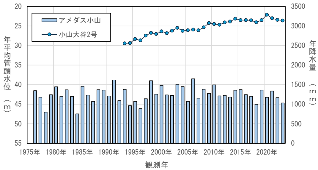
図4.3(32) 年平均地下水位の経年変化（小山大谷2号）
