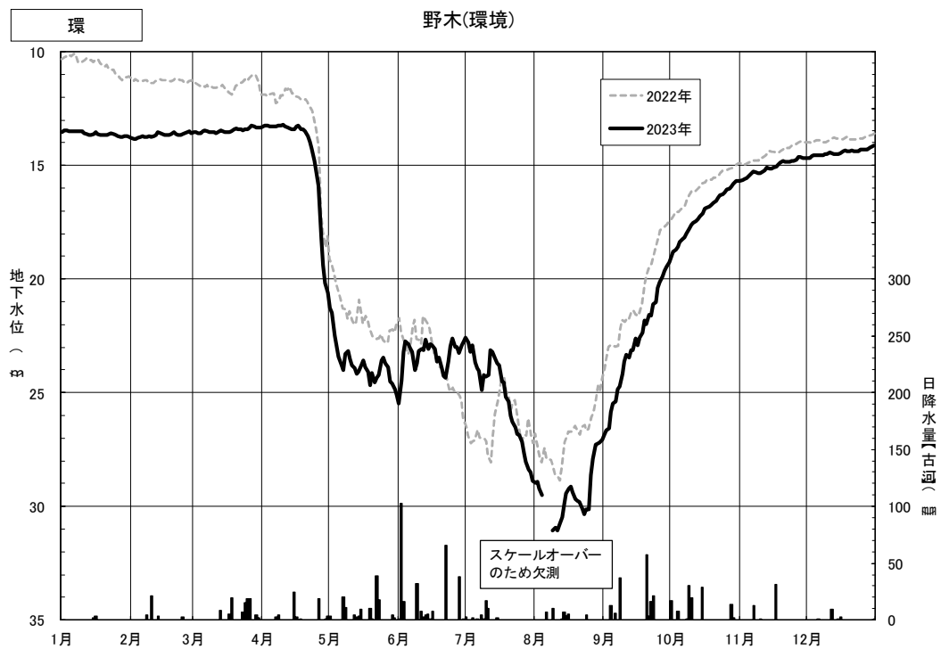
図4.3(61) 日地下水水位の年間変動（野木（環境））
