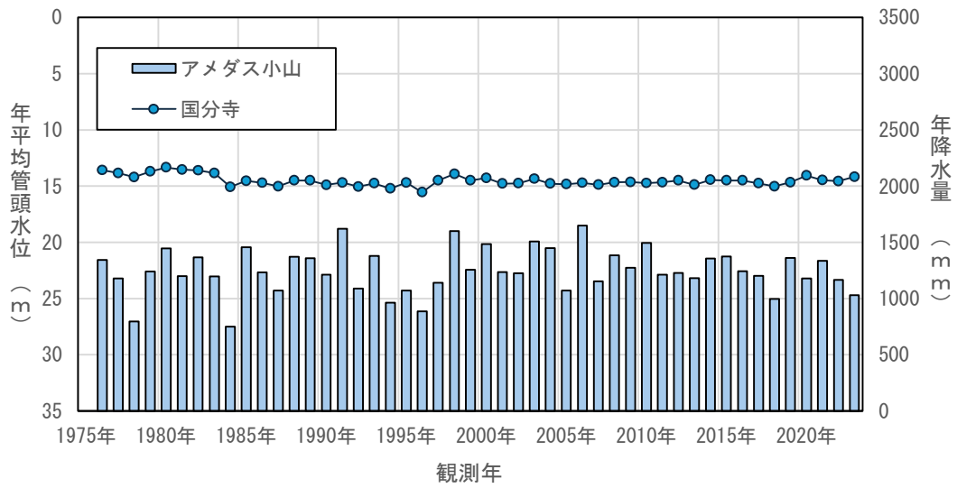
図4.3(63) 年平均地下水位の経年変化（国分寺）
