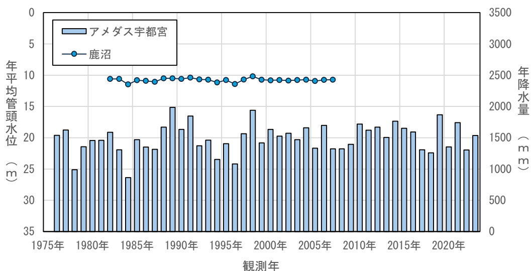
図4.3(94) 年平均地下水位の経年変化（鹿沼）
