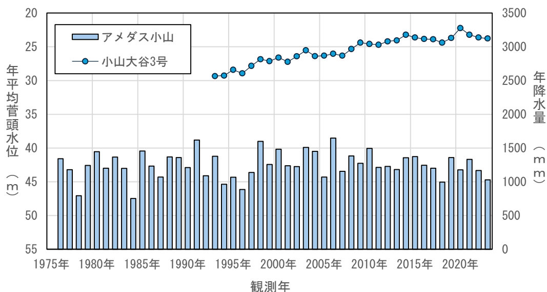
図4.3(34) 年平均地下水位の経年変化（小山大谷3号）
