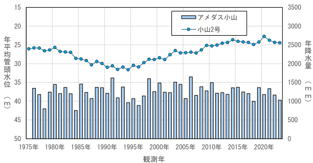
図 4.3(3) 年平均地下水水位の経年変化 (小山2号)
