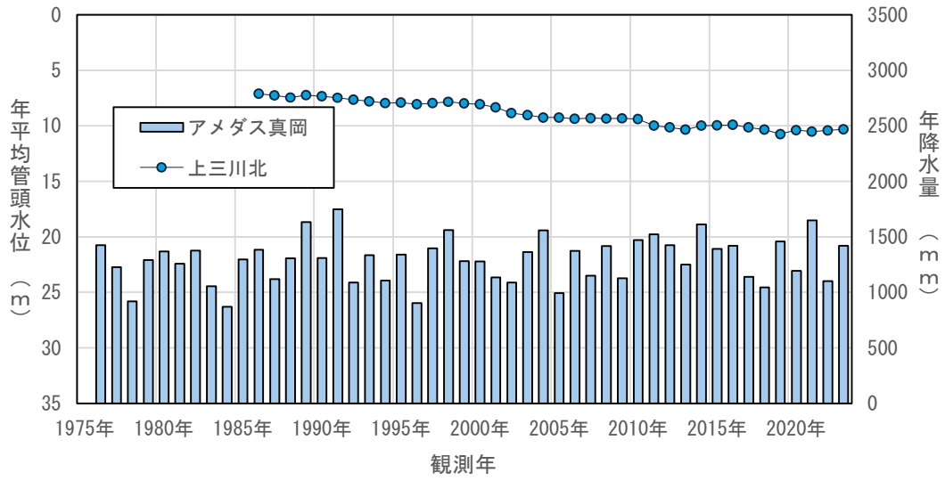
図4.3(79) 年平均地下水位の経年変化（上三川北）
