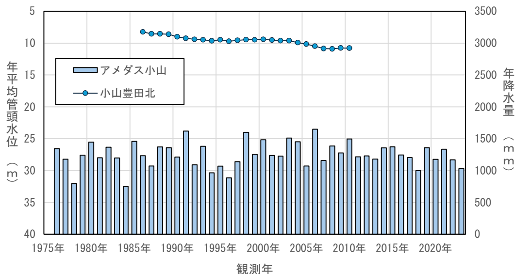
図4.3(7) 年平均地下水位の経年変化（小山豊田北）
