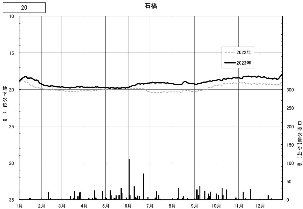
図4.3(66) 日地下水位の年間変動（石橋）
