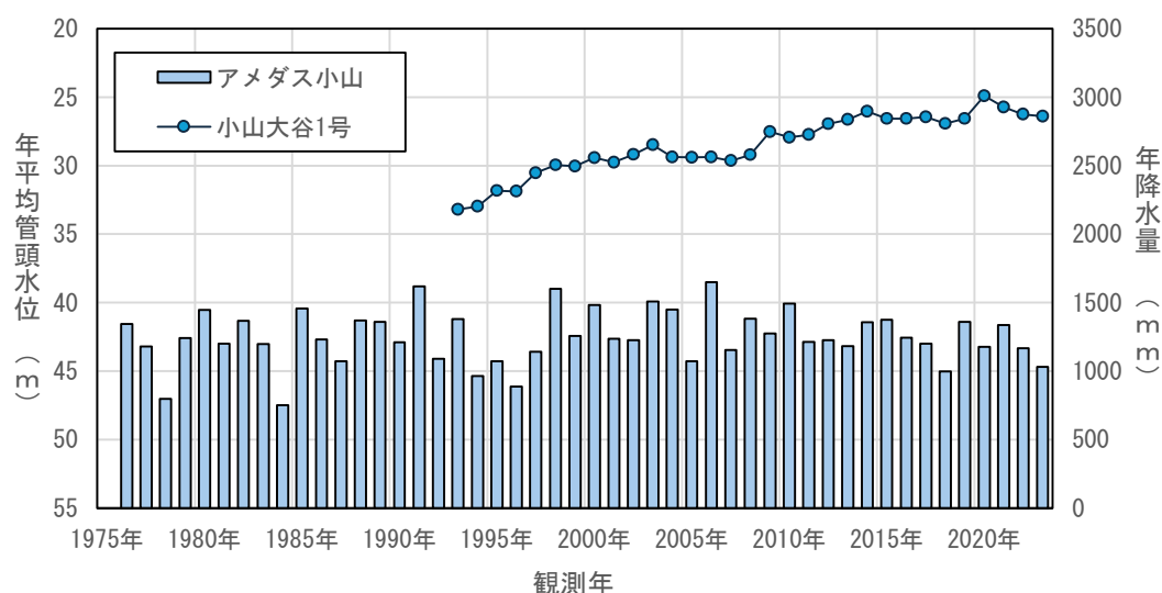
図4.3(30) 年平均地下水位の経年変化 (小山大谷1号)
