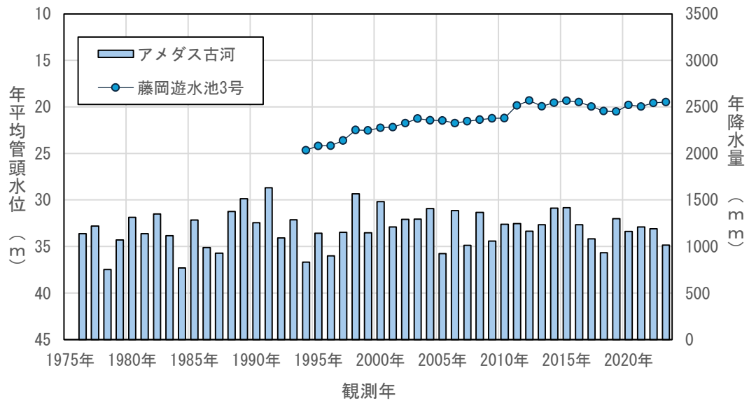
図4.3(40) 年平均地下水位の経年変化（藤岡遊水池3号）
