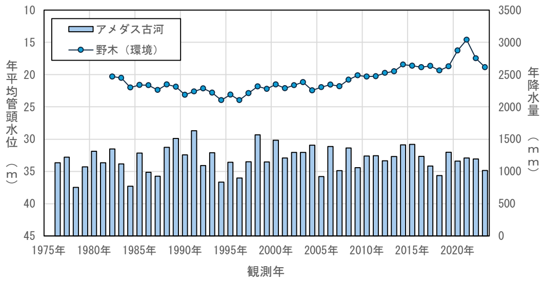
図4.3(60) 年平均地下水水位の経年変化（野木（環境））
