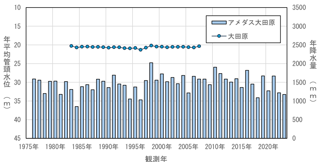
図4.3(98) 年平均地下水位の経年変化（大田原）
