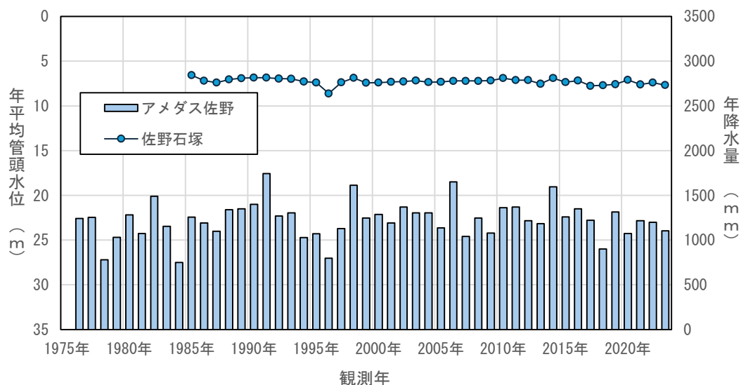
図4.3(22) 年平均地下水位の経年変化（佐野石塚）
