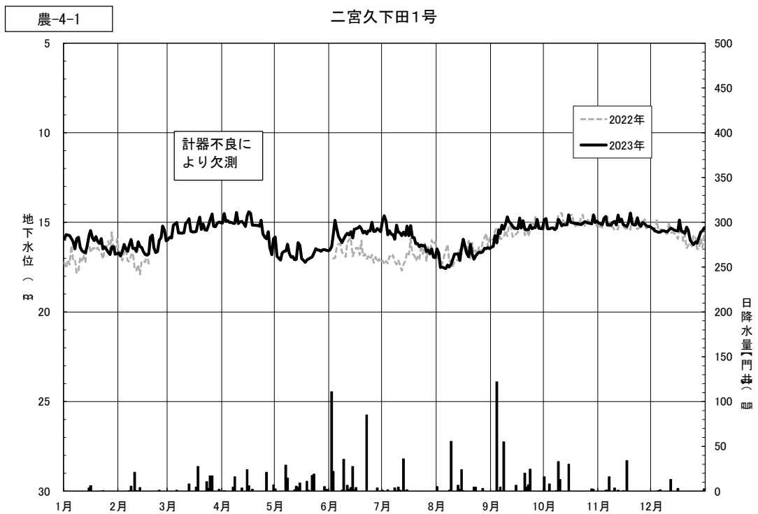
図4.3(87) 日地下水位の年間変動（二宮久下田1号）
