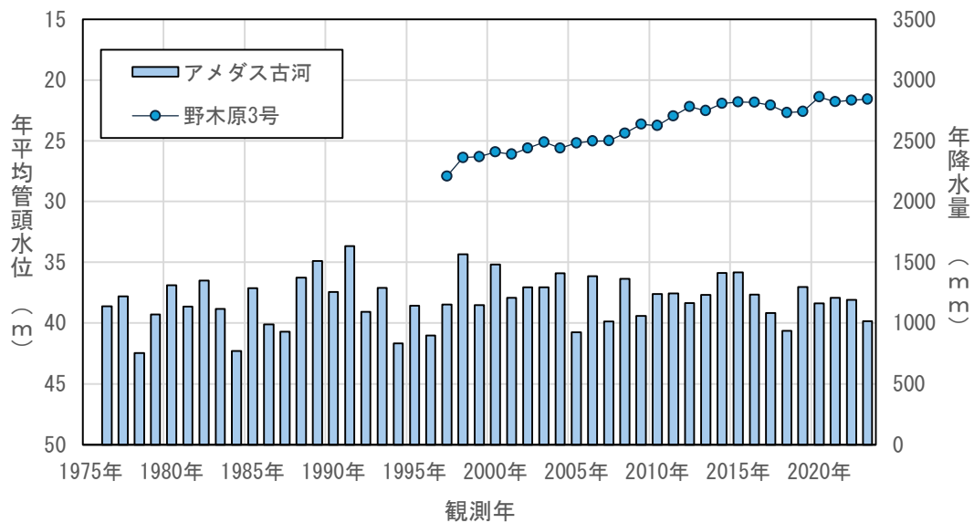
図4.3(46) 年平均地下水位の経年変化 (野木原3号)
