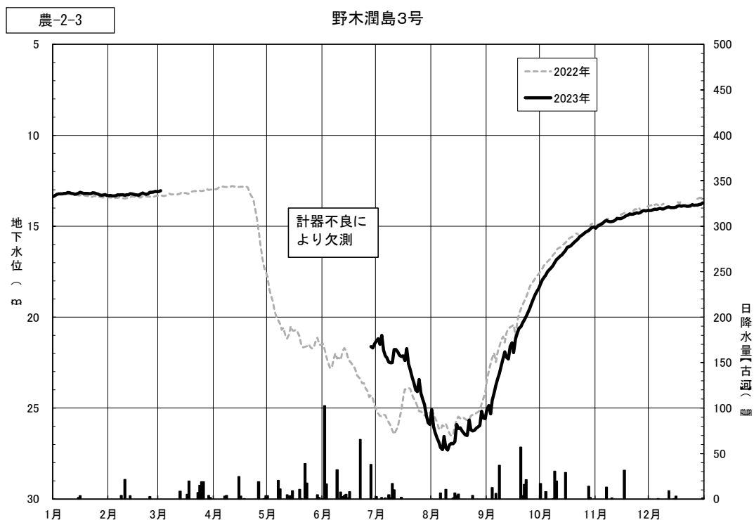
図4.3(55) 日地下水位の年間変動（野木潤島3号）
