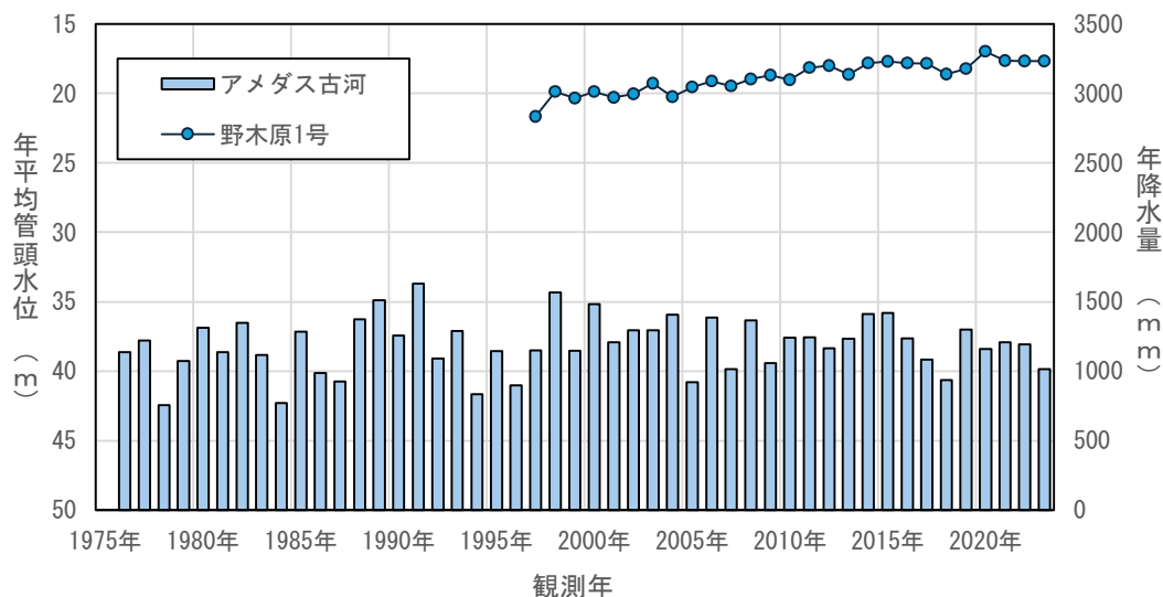
図4.3(42) 年平均地下水位の経年変化（野木原1号）
