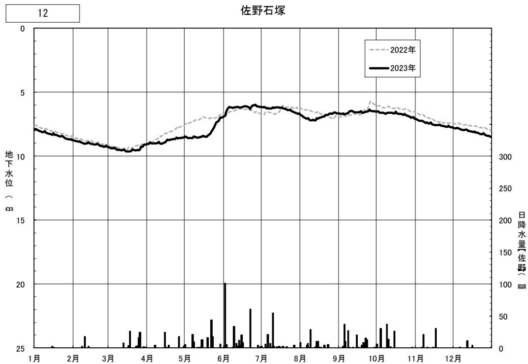
図4.3(23) 日地下水位の年間変動（佐野石塚）
