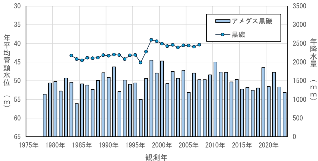
図4.3(99) 年平均地下水位の経年変化（黒磯）
