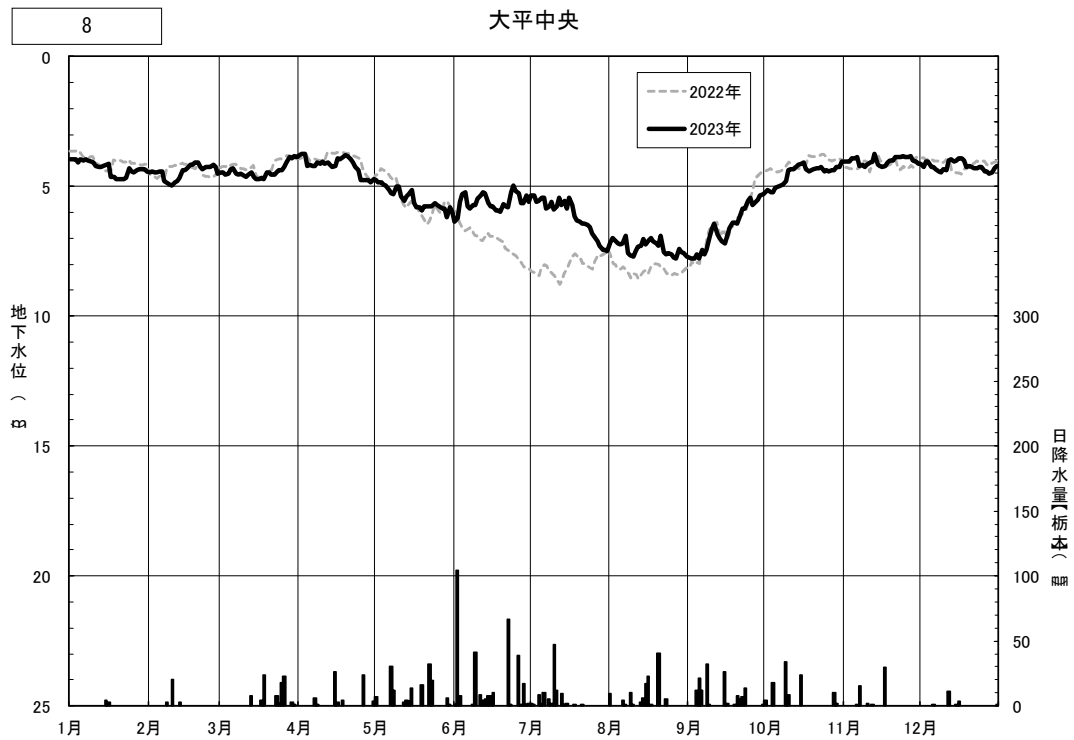
図4.3(17) 日地下水位の年間変動（大平中央）
