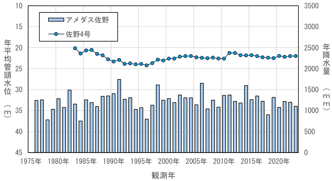
図4.3(20) 年平均地下水位の経年変化（佐野4号）
