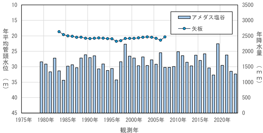
図4.3(97) 年平均地下水位の経年変化（矢板）
