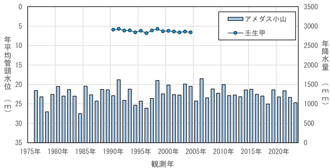
図4.3(85) 年平均地下水位の経年変化（壬生甲）
