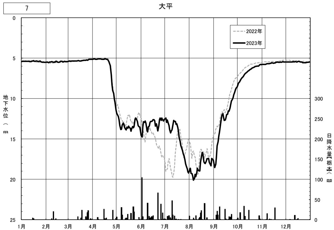
図4.3(15) 日地下水位の年間変動（大平）
