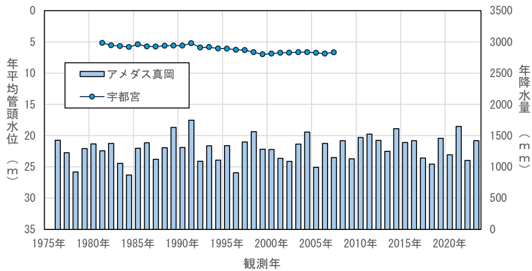
図4.3(83) 年平均地下水位の経年変化（宇都宮）
