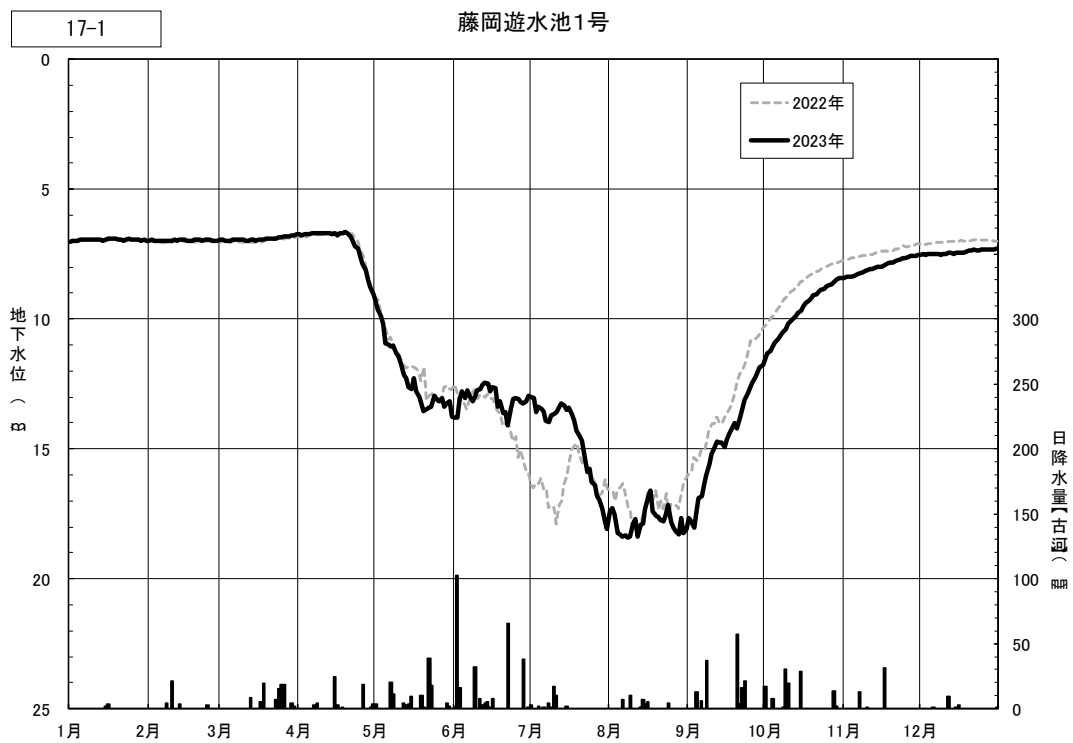
図4.3(37) 日地下水位の年間変動（藤岡遊水池1号）
