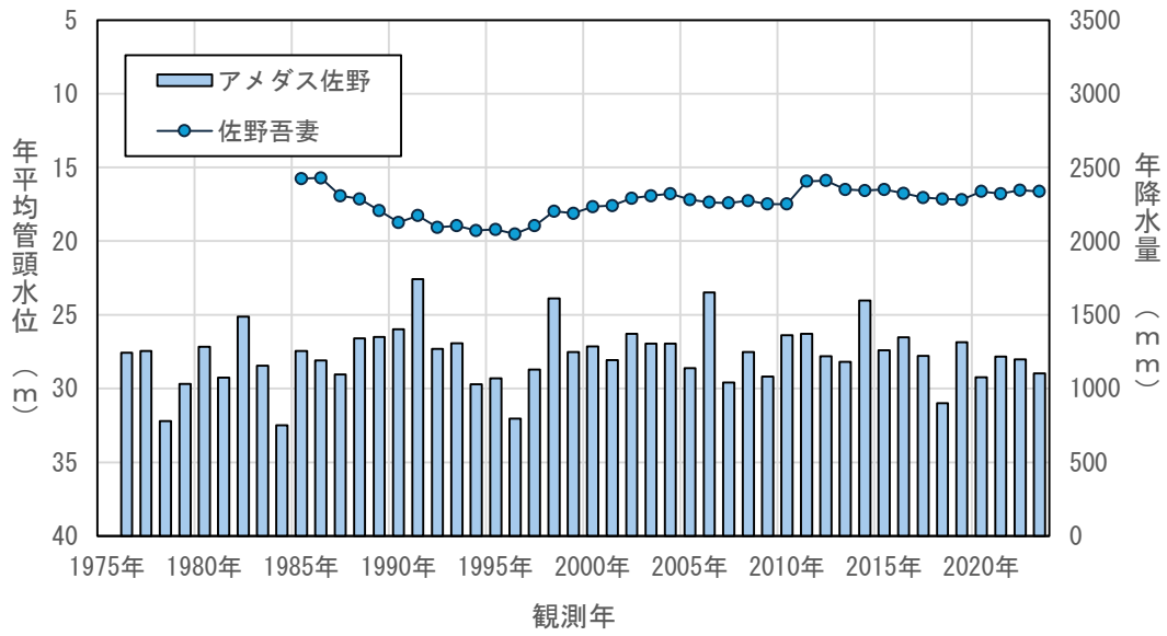
図4.3(24) 年平均地下水位の経年変化（佐野吾妻）
