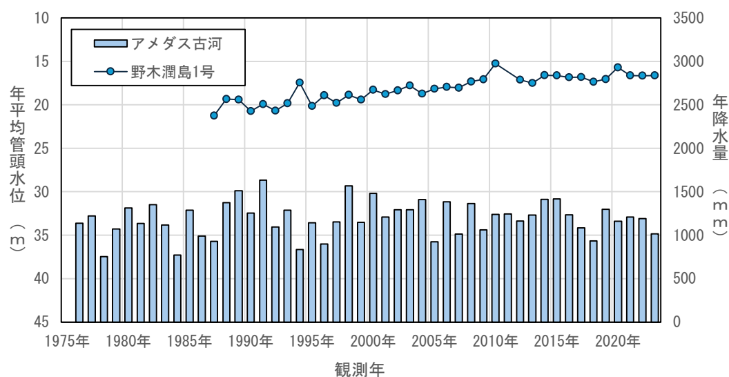
図4.3(50) 年平均地下水位の経年変化 (野木潤島1号)
