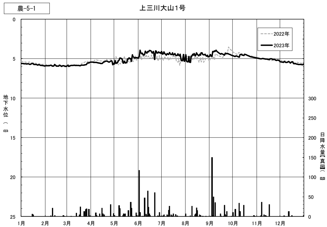
図4.3(91) 日地下水位の年間変動（上三川大山1号）
