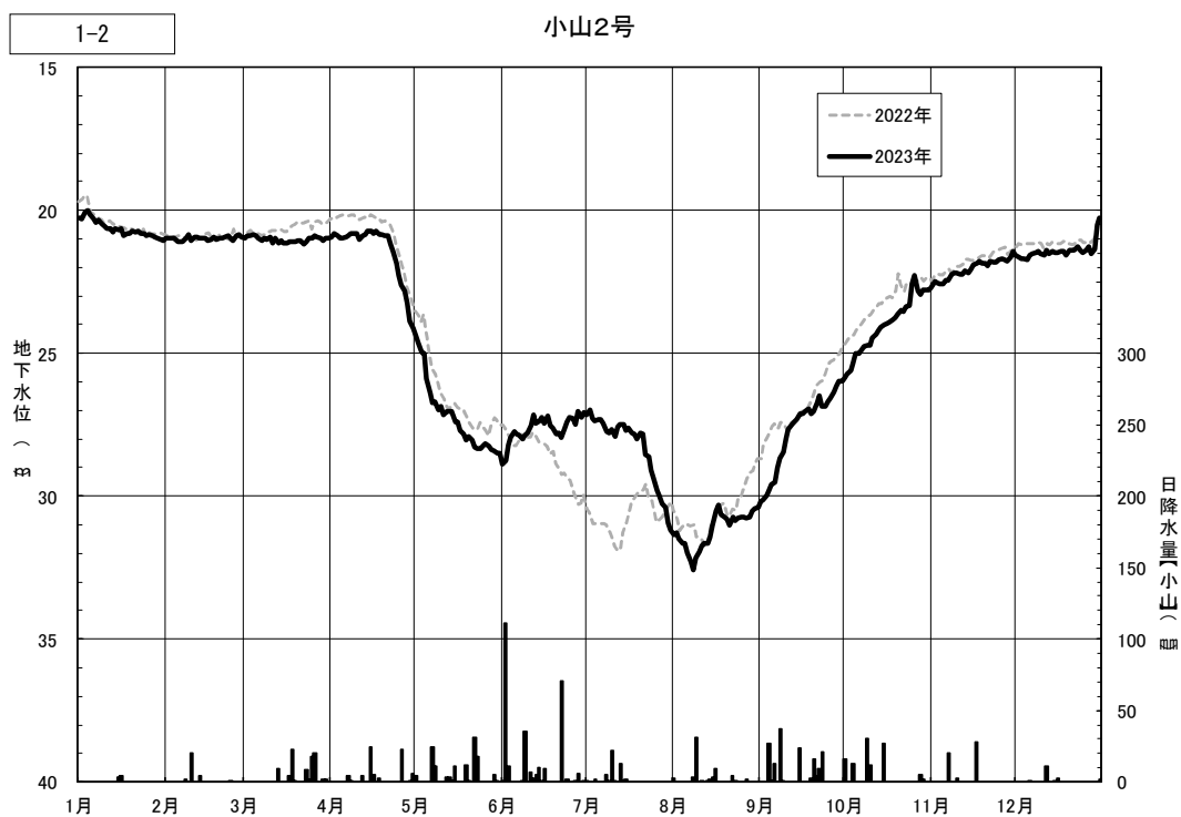
図 4.3(4) 日地下水水位の年間変動 (小山2号)
