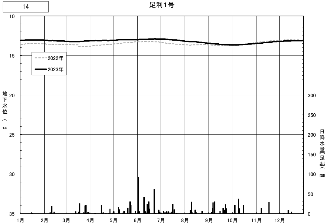
図4.3(27) 日地下水位の年間変動（足利1号）
