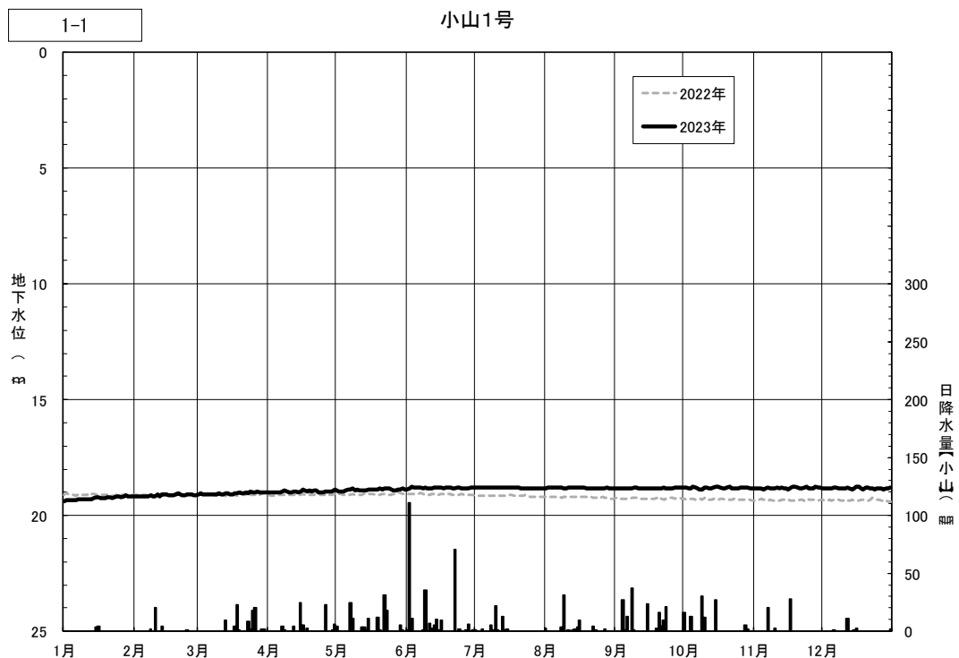
図 4.3(2) 日地下水位の年間変動 (小山1号)
