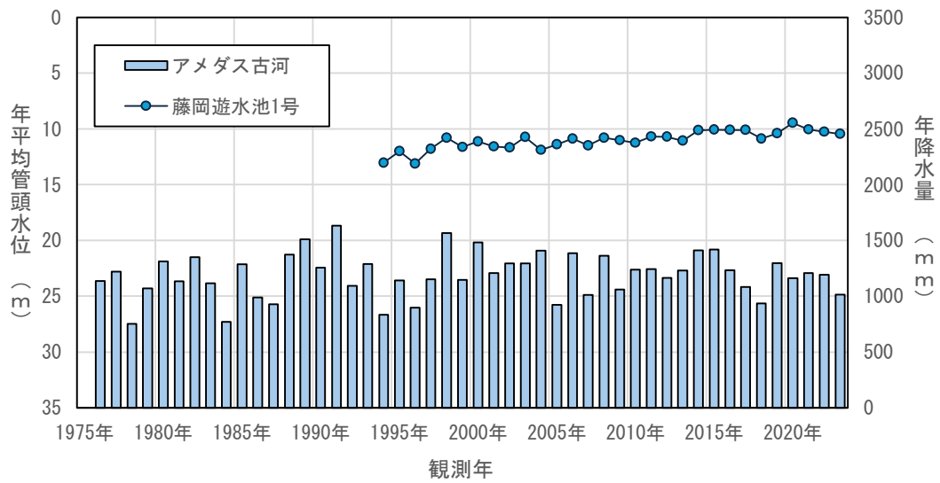
図4.3(36) 年平均地下水位の経年変化（藤岡遊水池1号）
