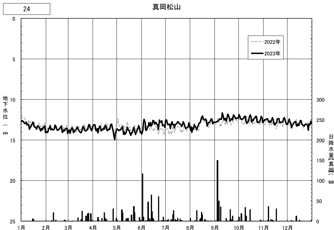
図4.3(74) 日地下水位の年間変動（真岡松山）
