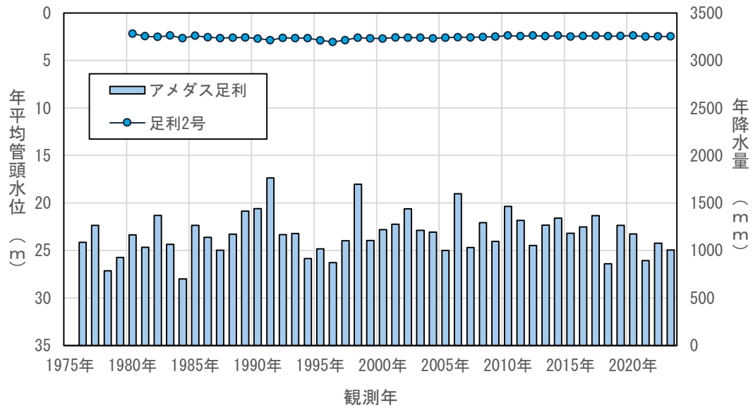
図4.3(28) 年平均地下水位の経年変化（足利2号）
