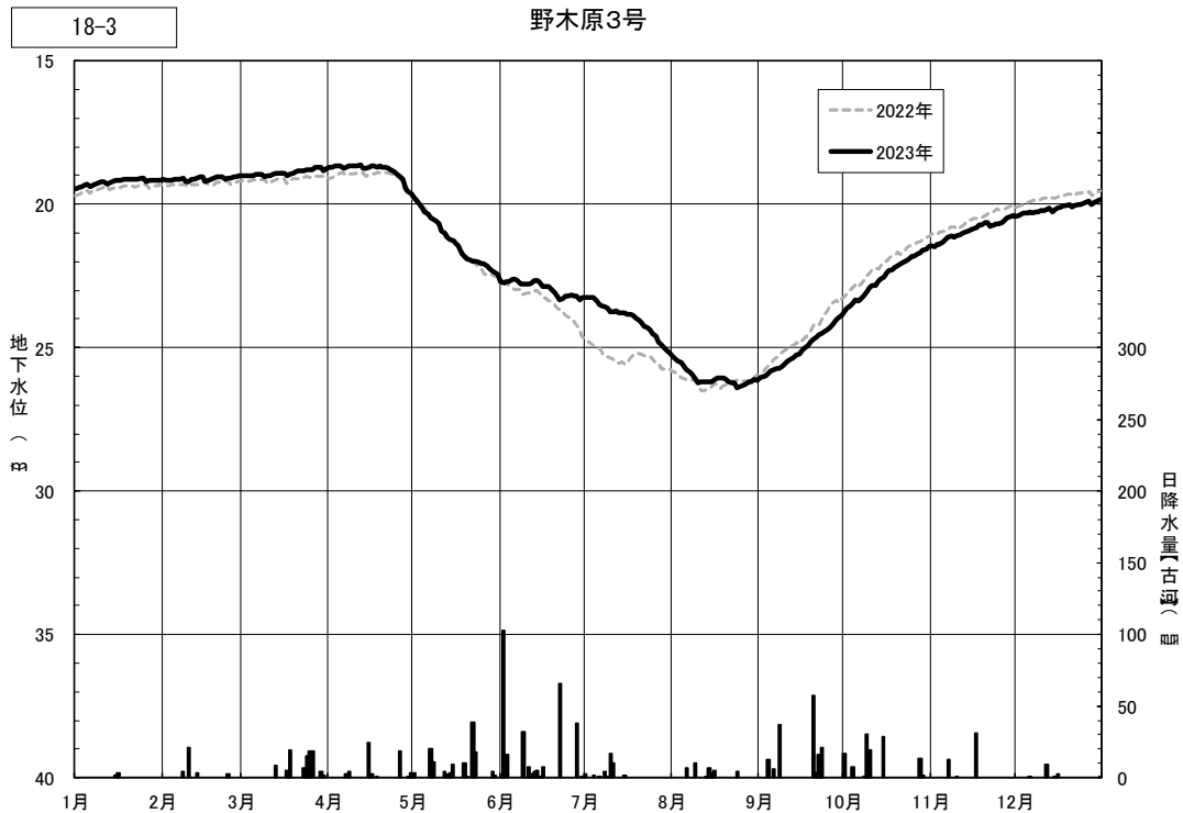
図4.3(47) 日地下水位の年間変動（野木原3号）
