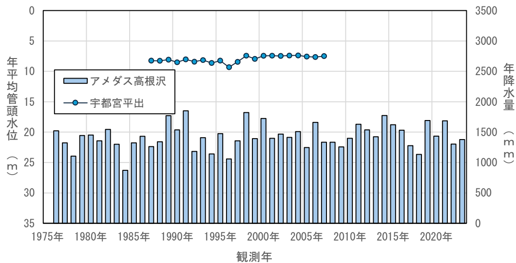
図4.3(84) 年平均地下水位の経年変化（宇都宮平出）
