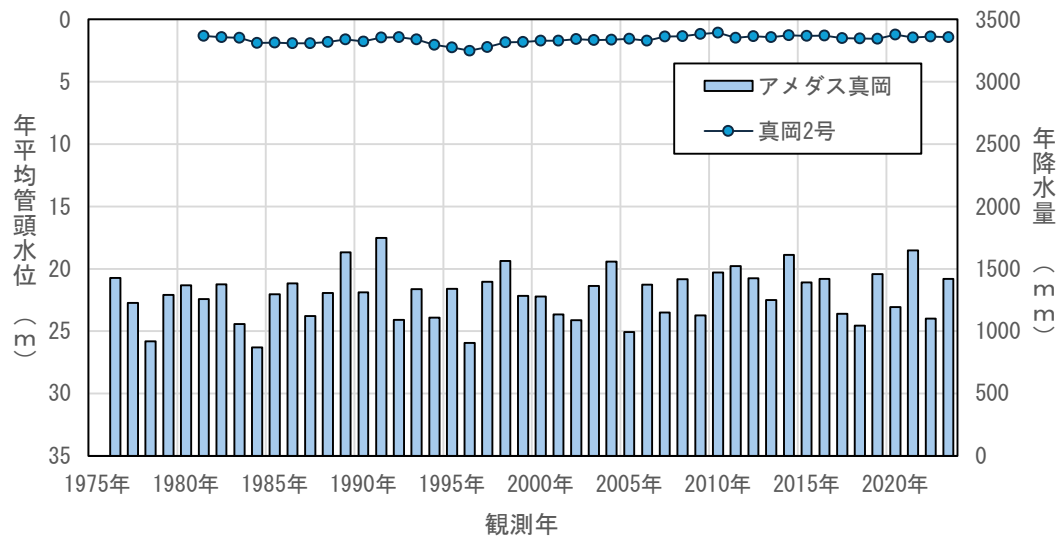
図4.3(71) 年平均地下水位の経年変化（真岡2号）
