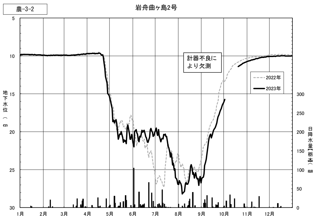
図4.3(59) 日地下水位の年間変動（岩舟曲ヶ島2号）
