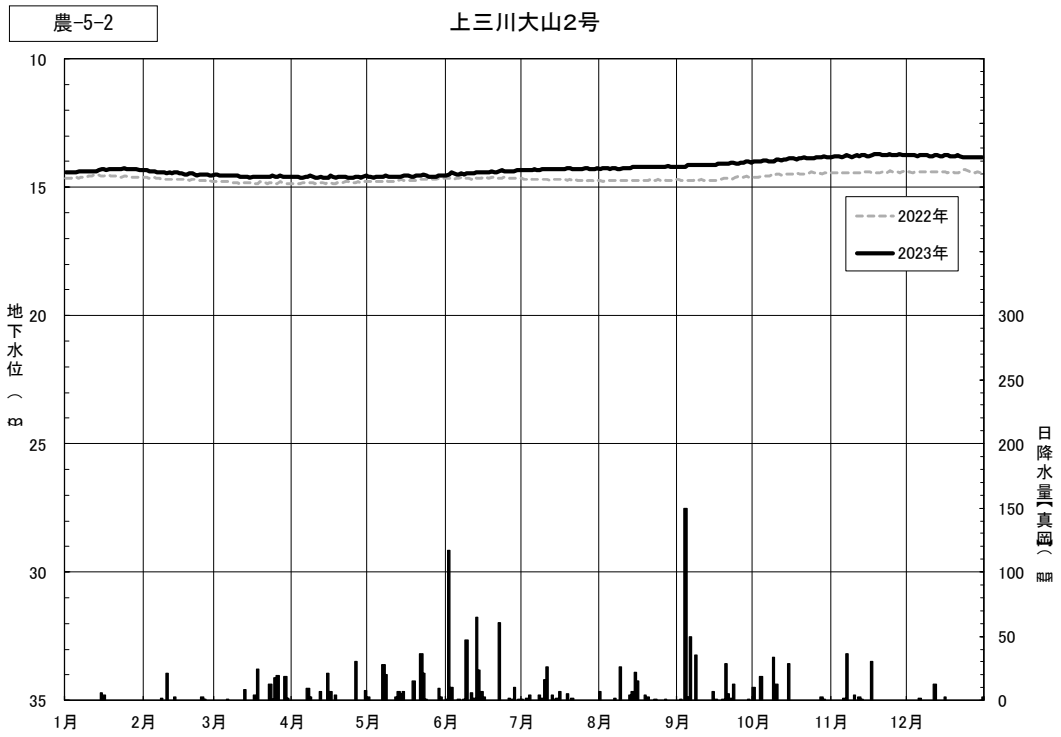
図4.3(93) 日地下水位の年間変動 (上三川大山2号)
