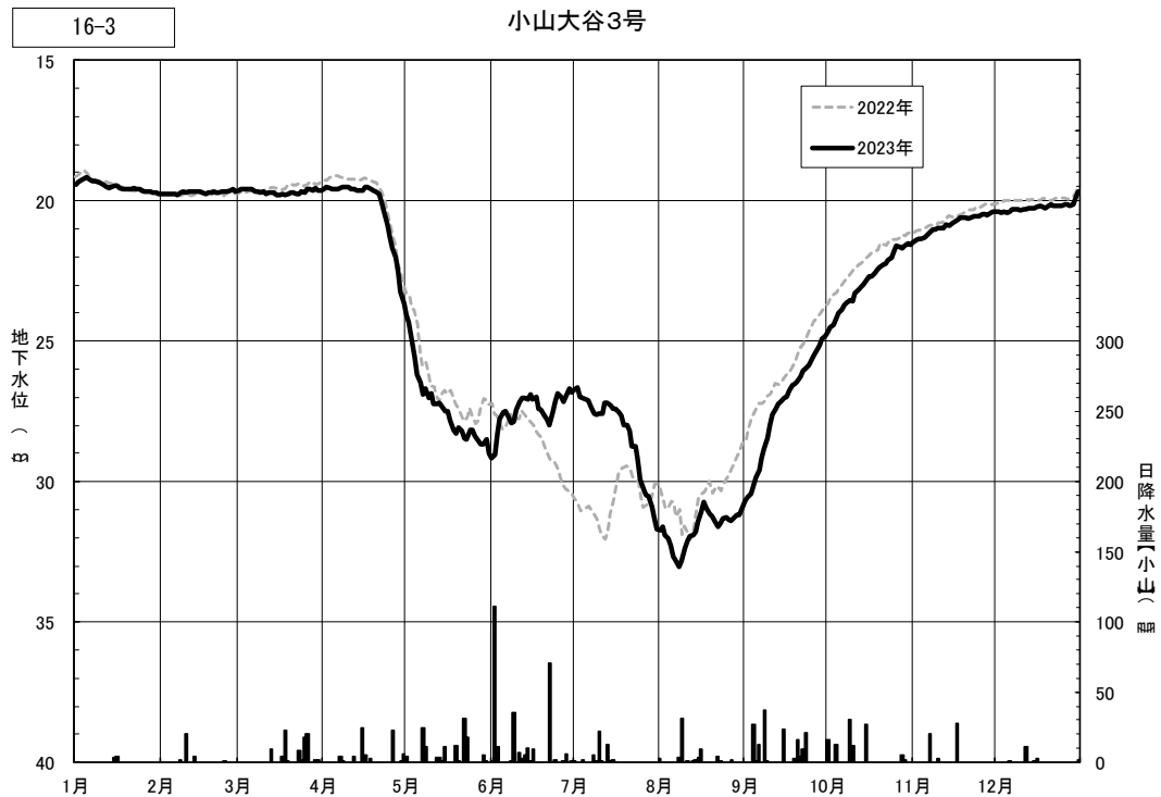
図4.3(35) 日地下水位の年間変動（小山大谷3号）
