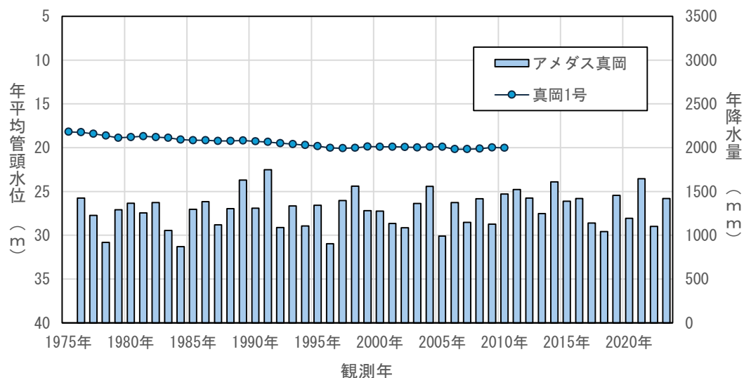
図4.3(70) 年平均地下水水位の経年変化（真岡1号）
