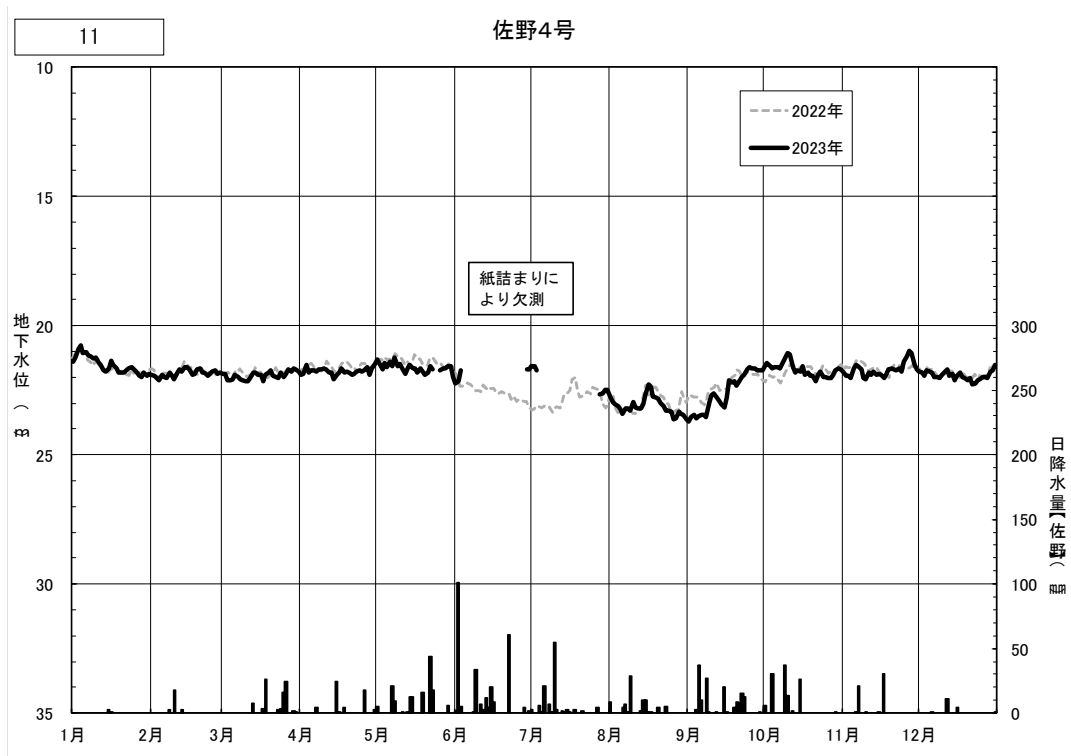
図4.3(21) 日地下水位の年間変動（佐野4号）
