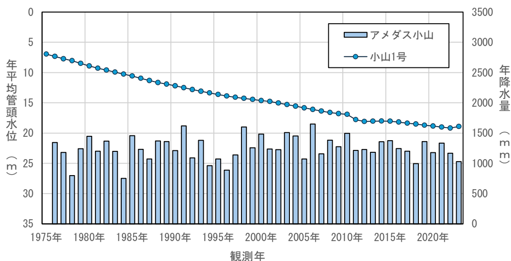
図 4.3(1) 年平均地下水位の経年変化（小山1号）
