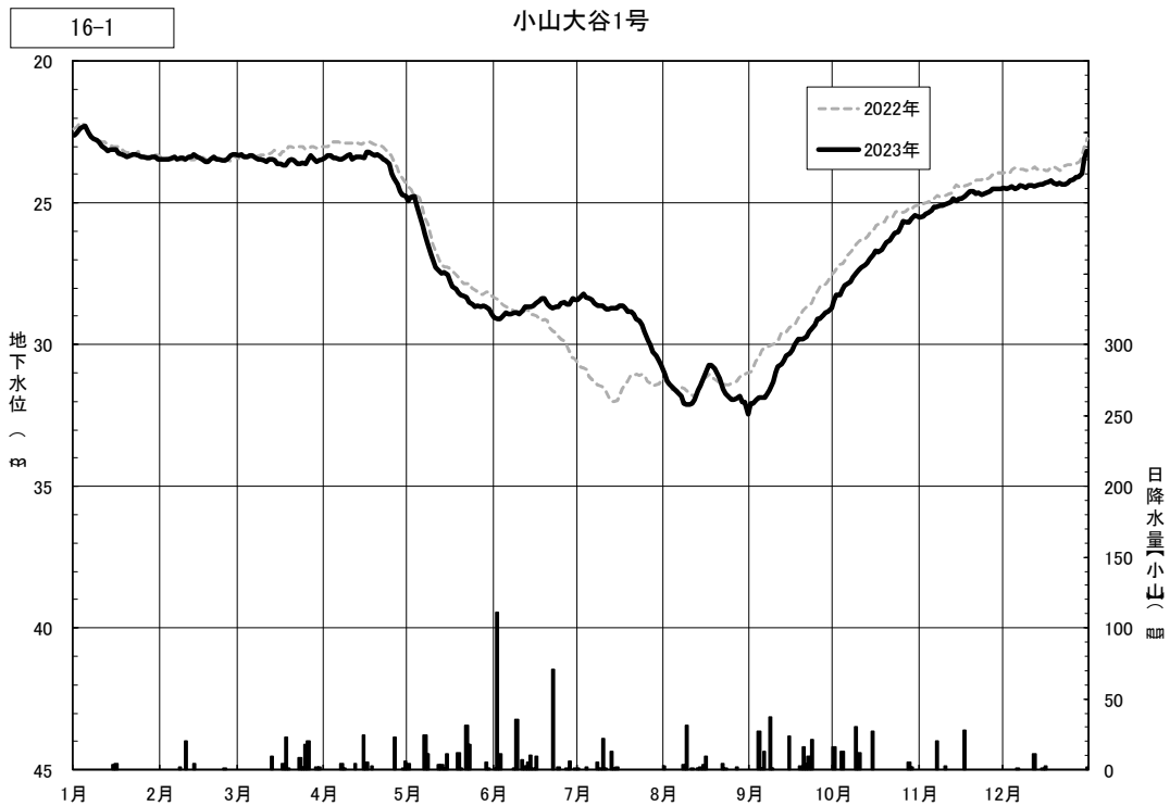
図4.3(31) 日地下水位の年間変動（小山大谷1号）
