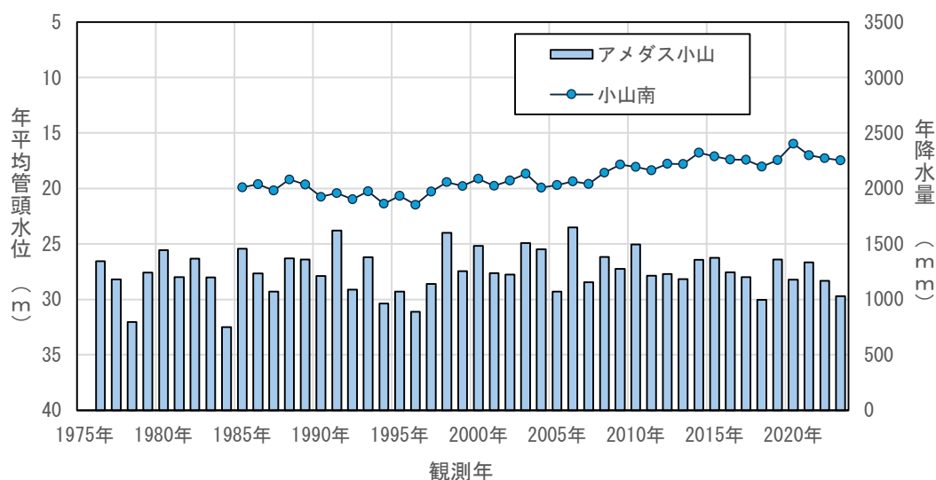
図 4.3(5) 年平均地下水位の経年変化 (小山南)
