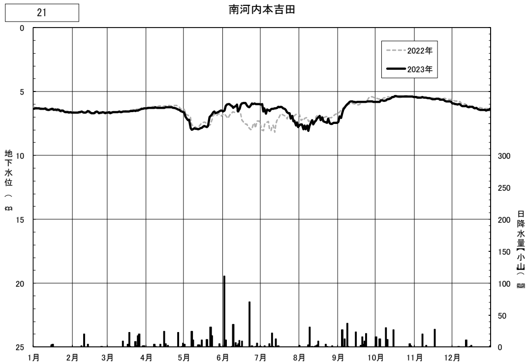
図4.3(68) 日地下水位の年間変動（南河内本吉田）
