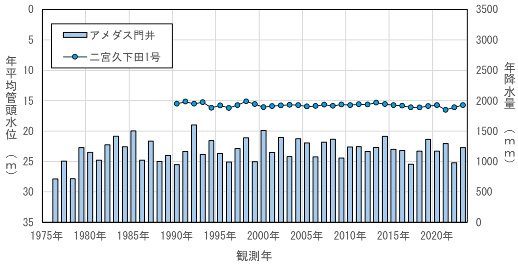
図4.3(86) 年平均地下水位の経年変化（二宮久下田1号）
