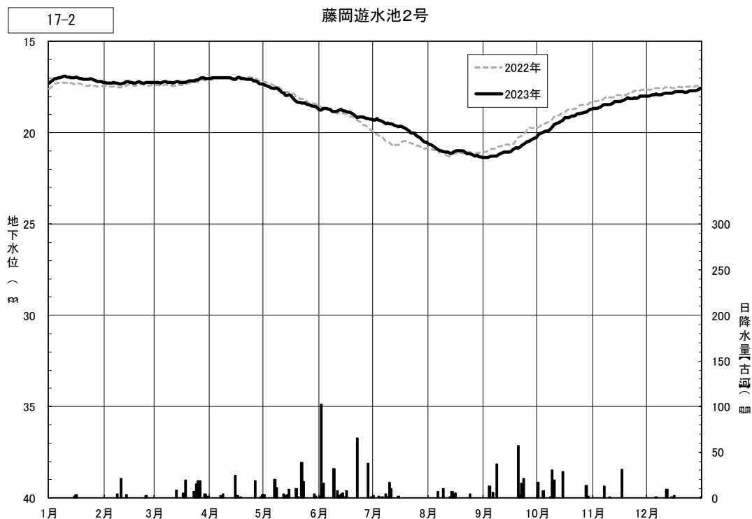
図4.3(39) 日地下水位の年間変動（藤岡遊水池2号）
