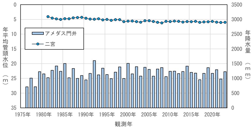
図4.3(75) 年平均地下水位の経年変化（二宮）
