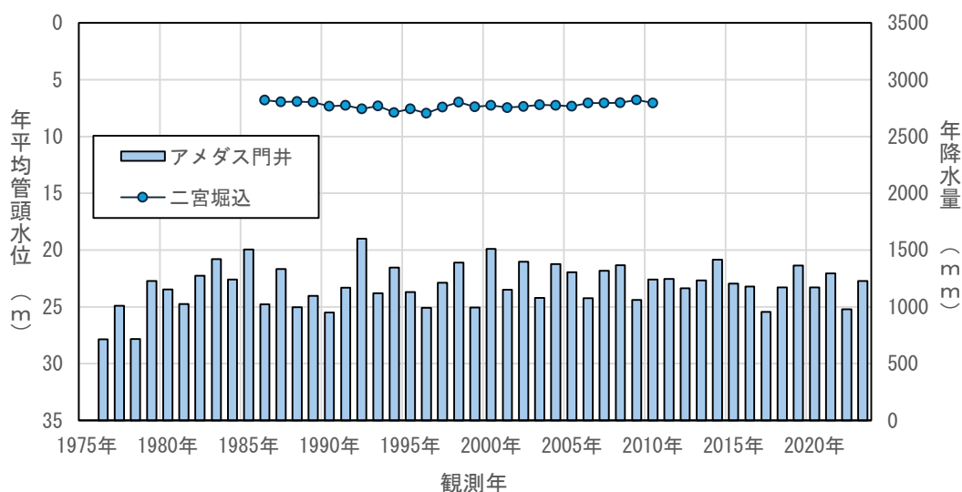
図4.3(77) 年平均地下水位の経年変化（二宮堀込）
