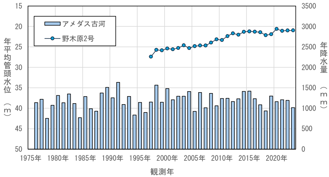
図4.3(44) 年平均地下水位の経年変化（野木原2号）
