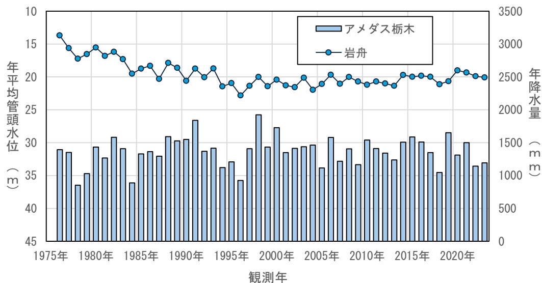
図4.3(10) 年平均地下水位の経年変化（岩舟）
