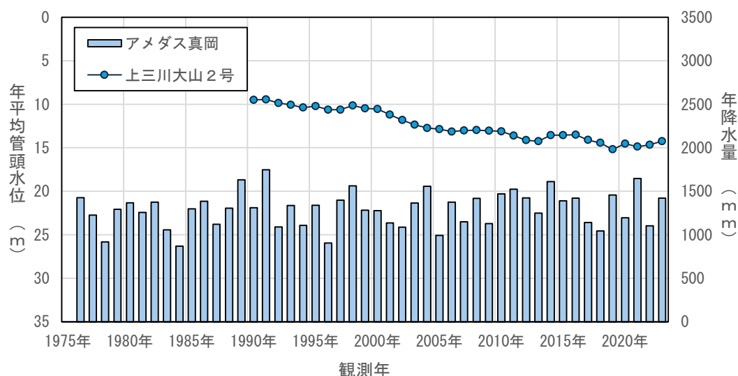
図4.3 (92) 年平均地下水位の経年変化（上三川大山2号）
