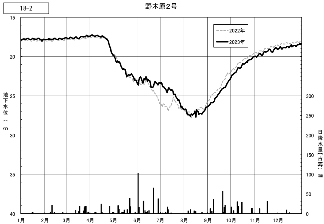
図4.3(45) 日地下水位の年間変動（野木原2号）
