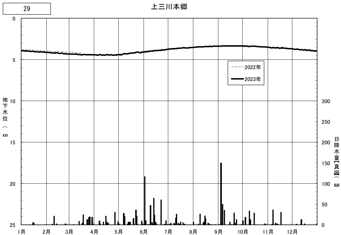
図 4.3(82) 日地下水位の年間変動（上三川本郷）
