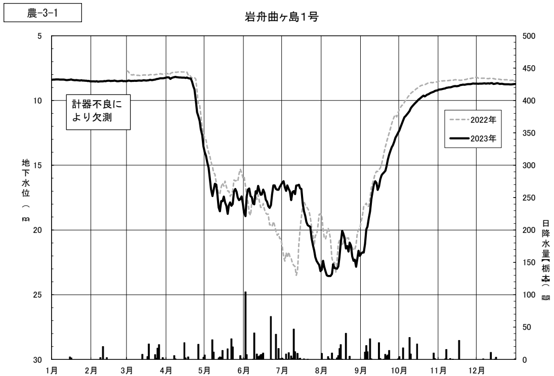
図4.3(57) 日地下水位の年間変動（岩舟曲ヶ島1号）
