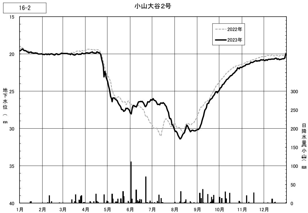
図4.3(33) 日地下水位の年間変動（小山大谷2号）
