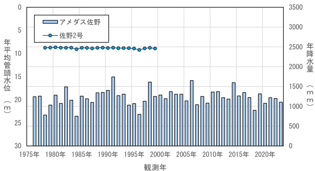
図4.3(18) 年平均地下水位の経年変化（佐野2号）
