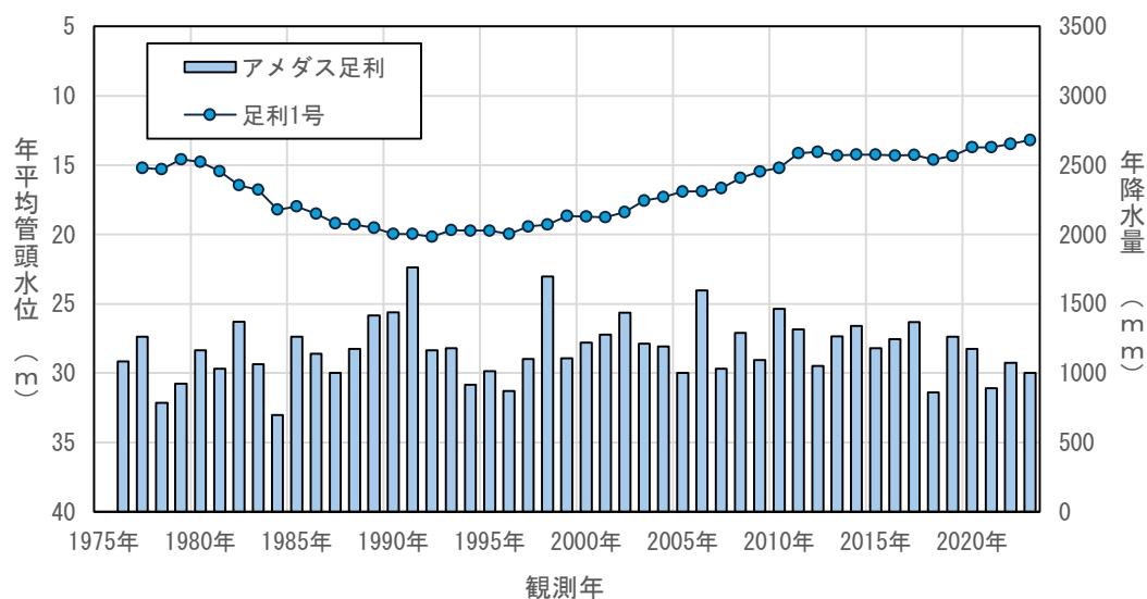
図4.3(26) 年平均地下水位の経年変化（足利1号）
