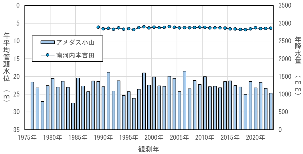
図4.3(67) 年平均地下水位の経年変化（南河内本吉田）
