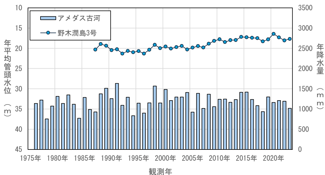
図4.3(54) 年平均地下水位の経年変化 (野木潤島3号)
