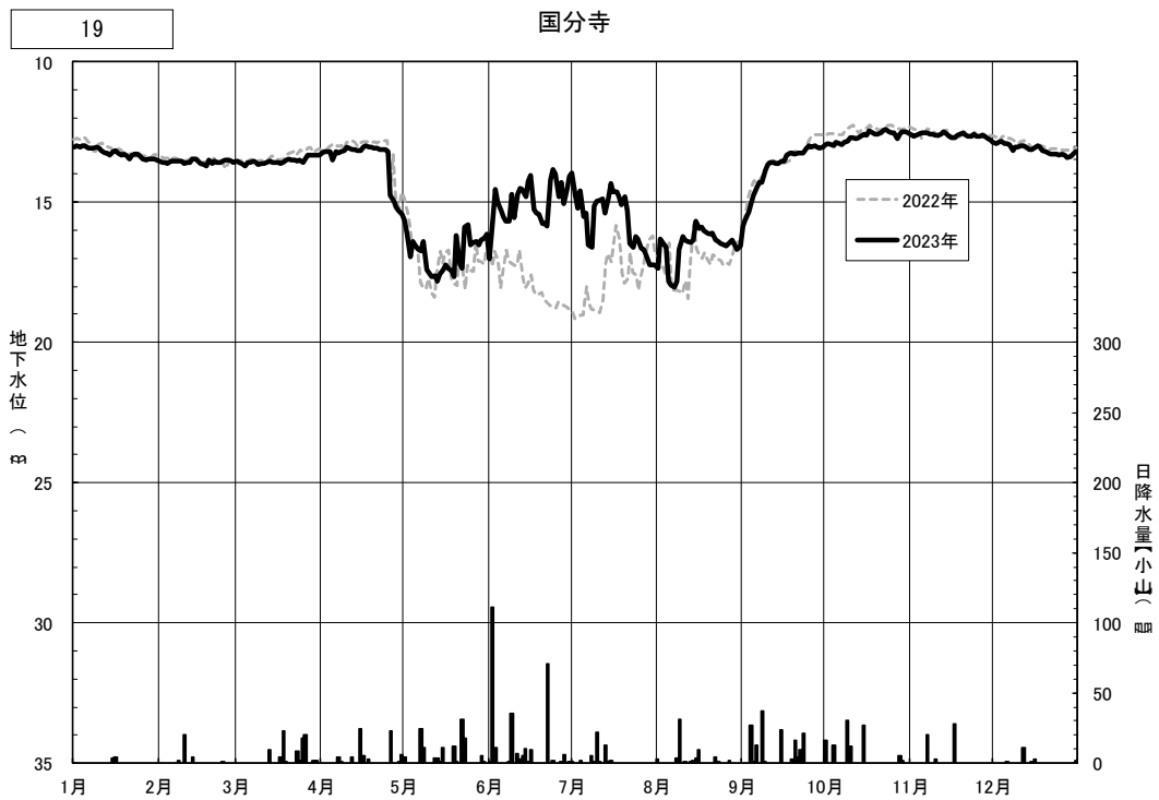
図4.3(64) 日地下水位の年間変動（国分寺）
