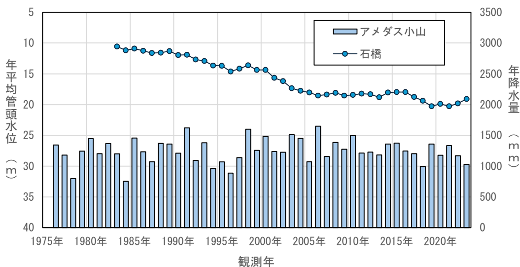
図4.3(65) 年平均地下水位の経年変化（石橋）
