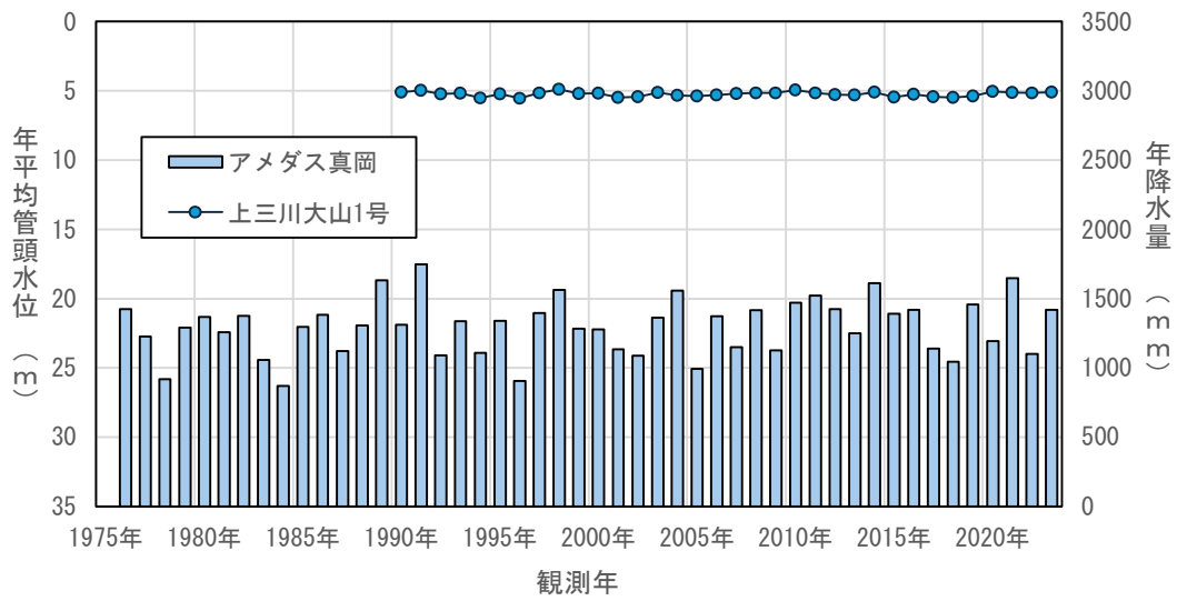
図4.3(90) 年平均地下水位の経年変化（上三川大山1号）
