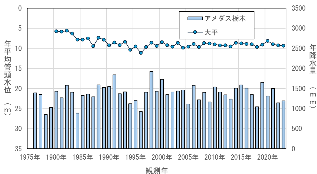
図4.3(14) 年平均地下水位の経年変化 (大平)
