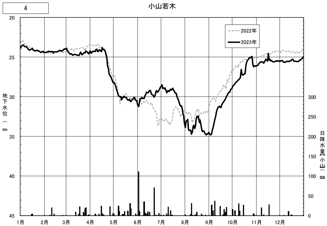
図4.3(9) 日地下水位の年間変動 (小山若木)
