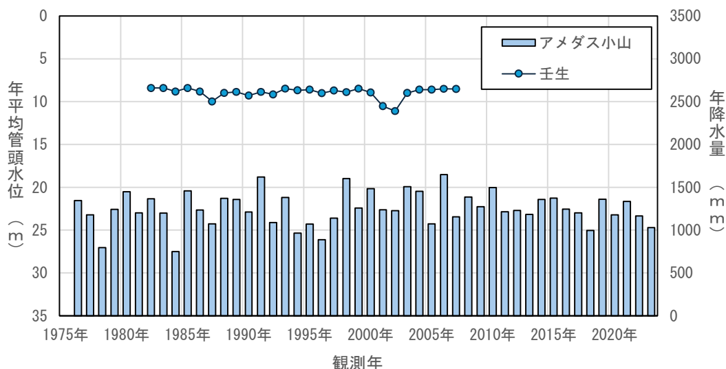
図4.3(69) 年平均地下水位の経年変化（壬生）
