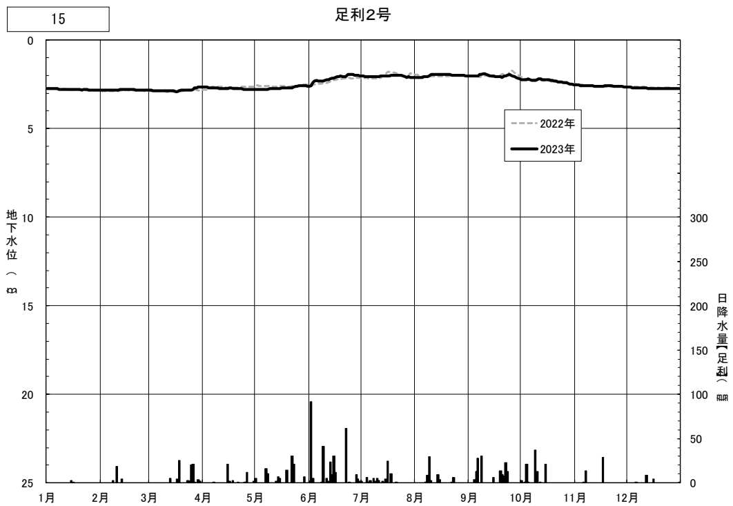
図4.3(29) 日地下水位の年間変動（足利2号）
