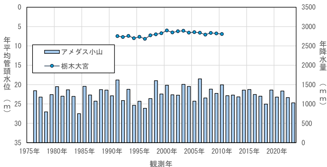
図4.3(62) 年平均地下水位の経年変化（栃木大宮）
