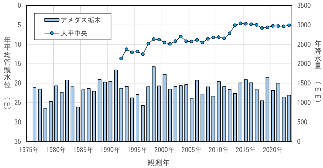
図4.3(16) 年平均地下水位の経年変化（大平中央）
