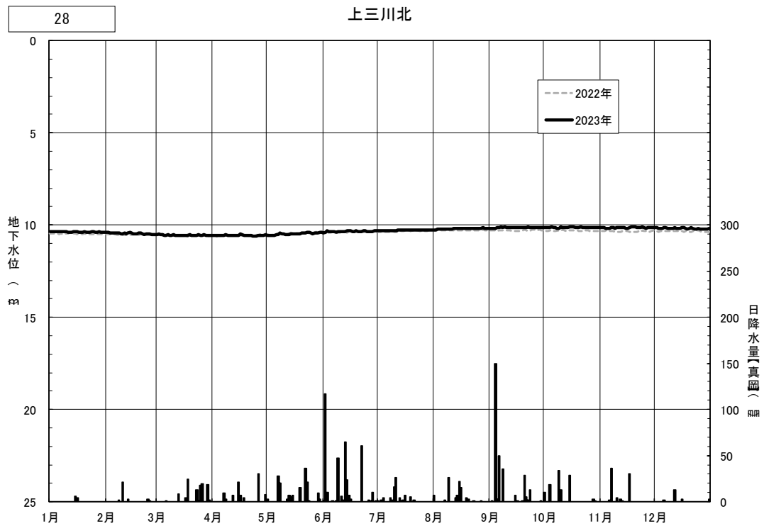
図4.3(80) 日地下水位の年間変動（上三川北）
