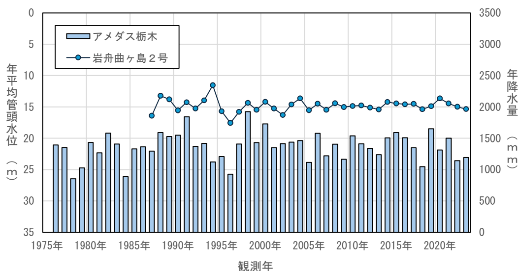
図4.3(58) 年平均地下水位の経年変化 (岩舟曲ヶ島2号)
