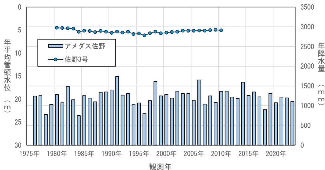
図4.3(19) 年平均地下水位の経年変化（佐野3号）
