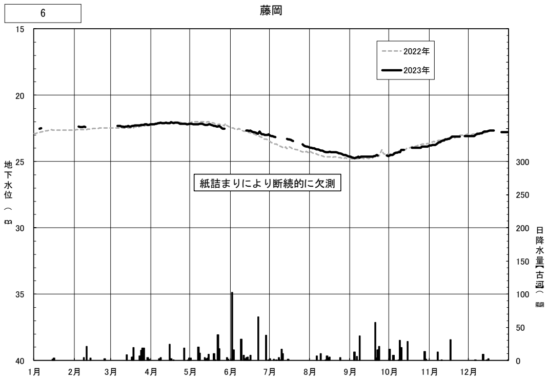
図4.3(13) 日地下水位の年間変動（藤岡）
