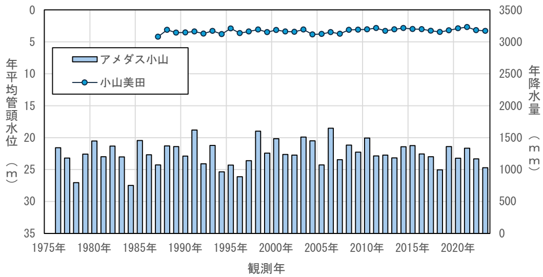
図4.3(48) 年平均地下水位の経年変化（小山美田）
