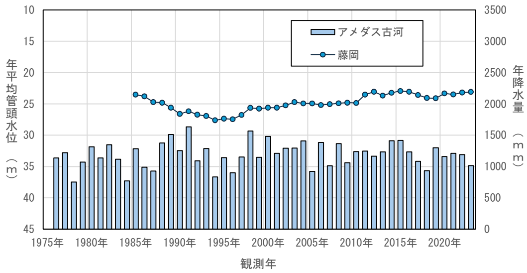
図4.3(12) 年平均地下水位の経年変化（藤岡）
