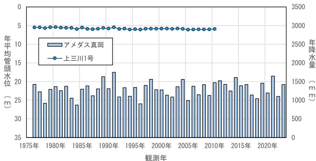
図4.3(78) 年平均地下水位の経年変化（上三川1号）
