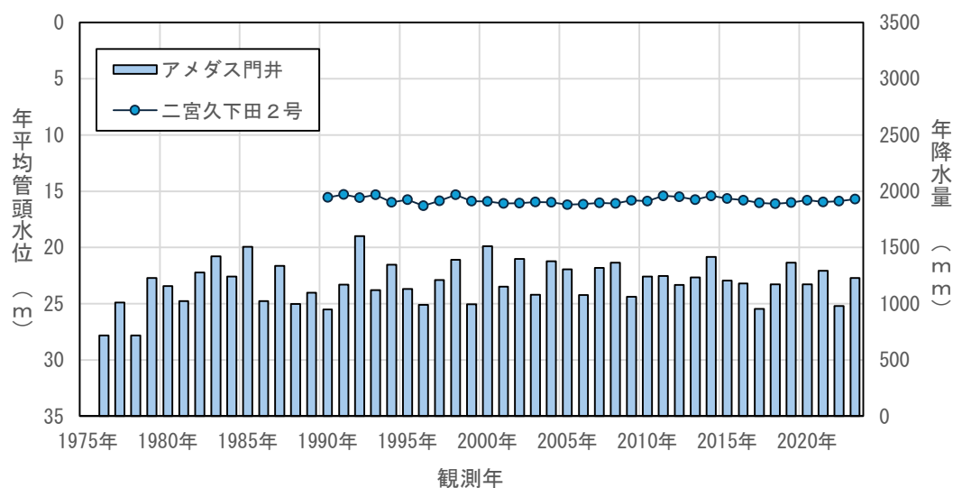
図4.3(88) 年平均地下水位の経年変化（二宮久下田 2号）
