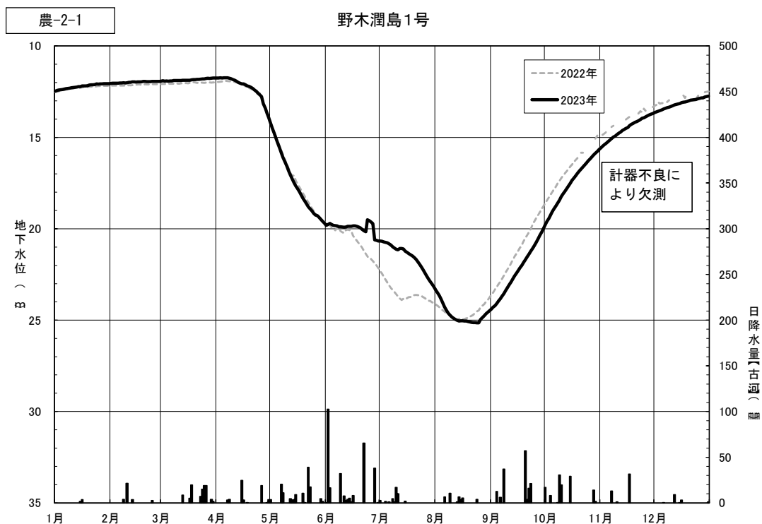
図 4.3(51) 日地下水位の年間変動（野木潤島 1 号）
