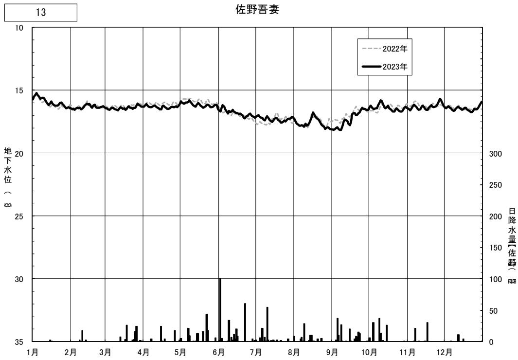
図4.3(25) 日地下水位の年間変動（佐野吾妻）
