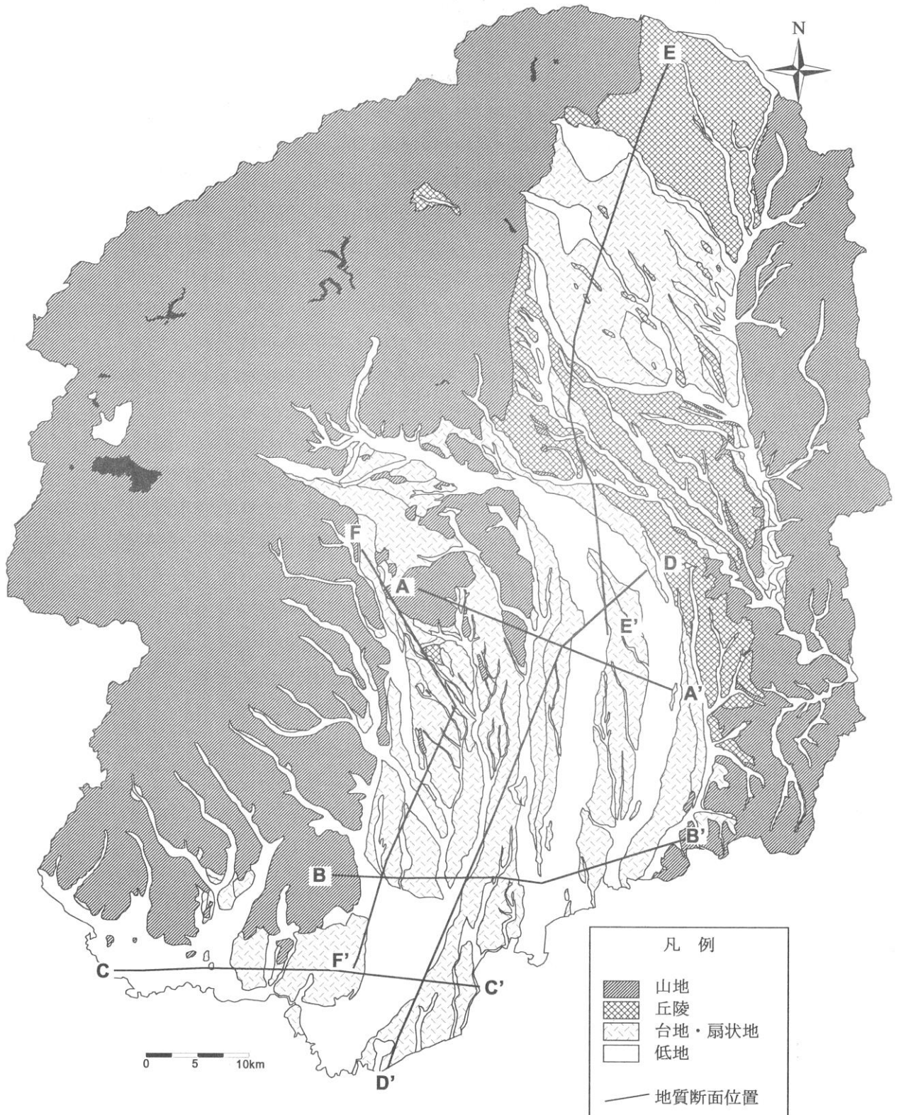
图-8 水理地質断面位置图
