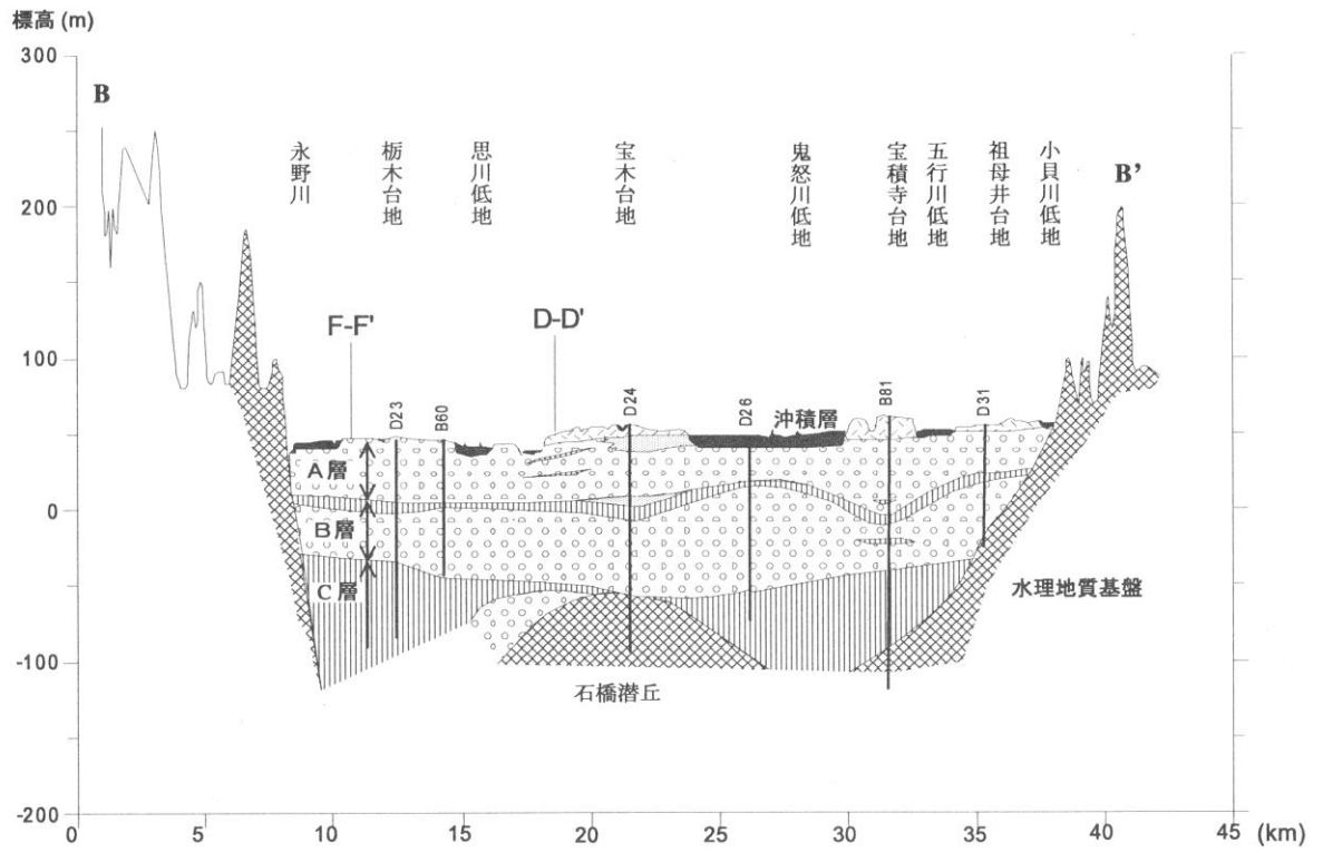
図-10 水理地質断面図 (B-B' 断面、C-C' 断面)
