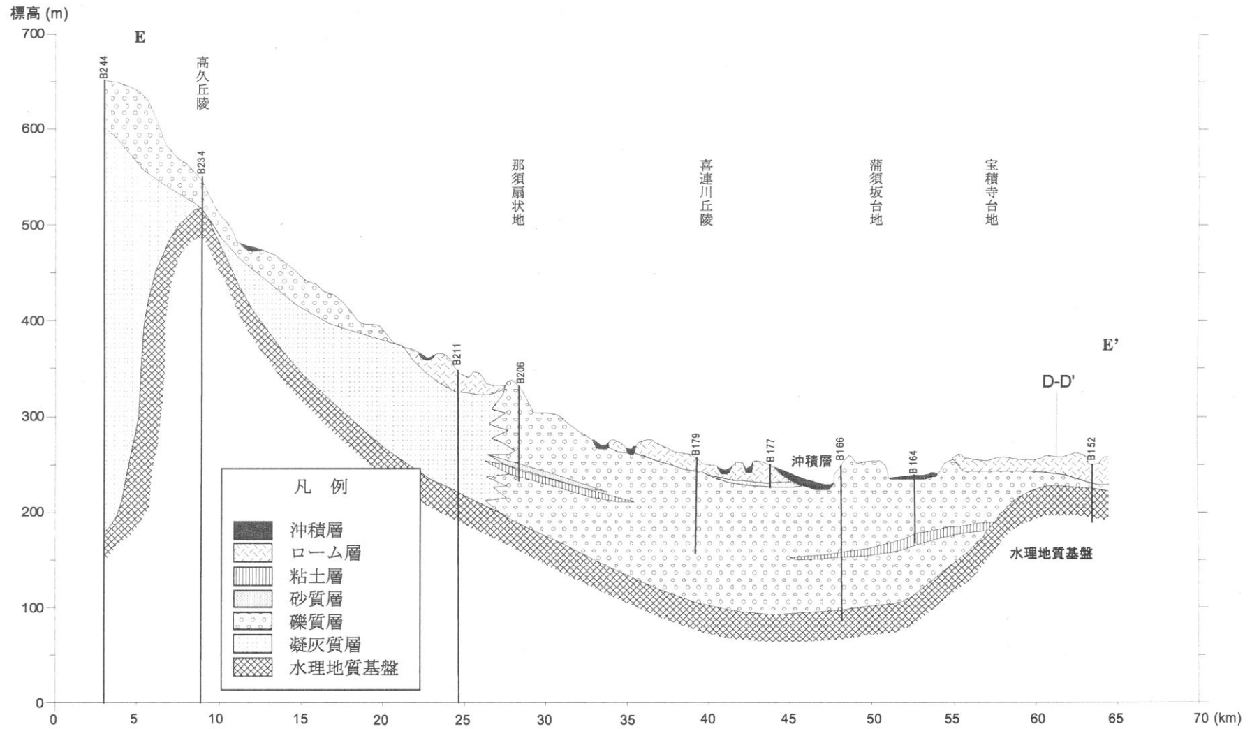
図-12 水理地質断面図 (E-E' 断面)
