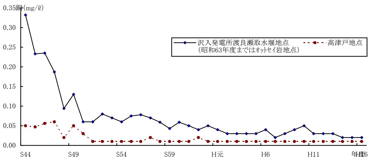
図2 - 6 渡良瀬川のかんがい期平均値経年変化(銅)
